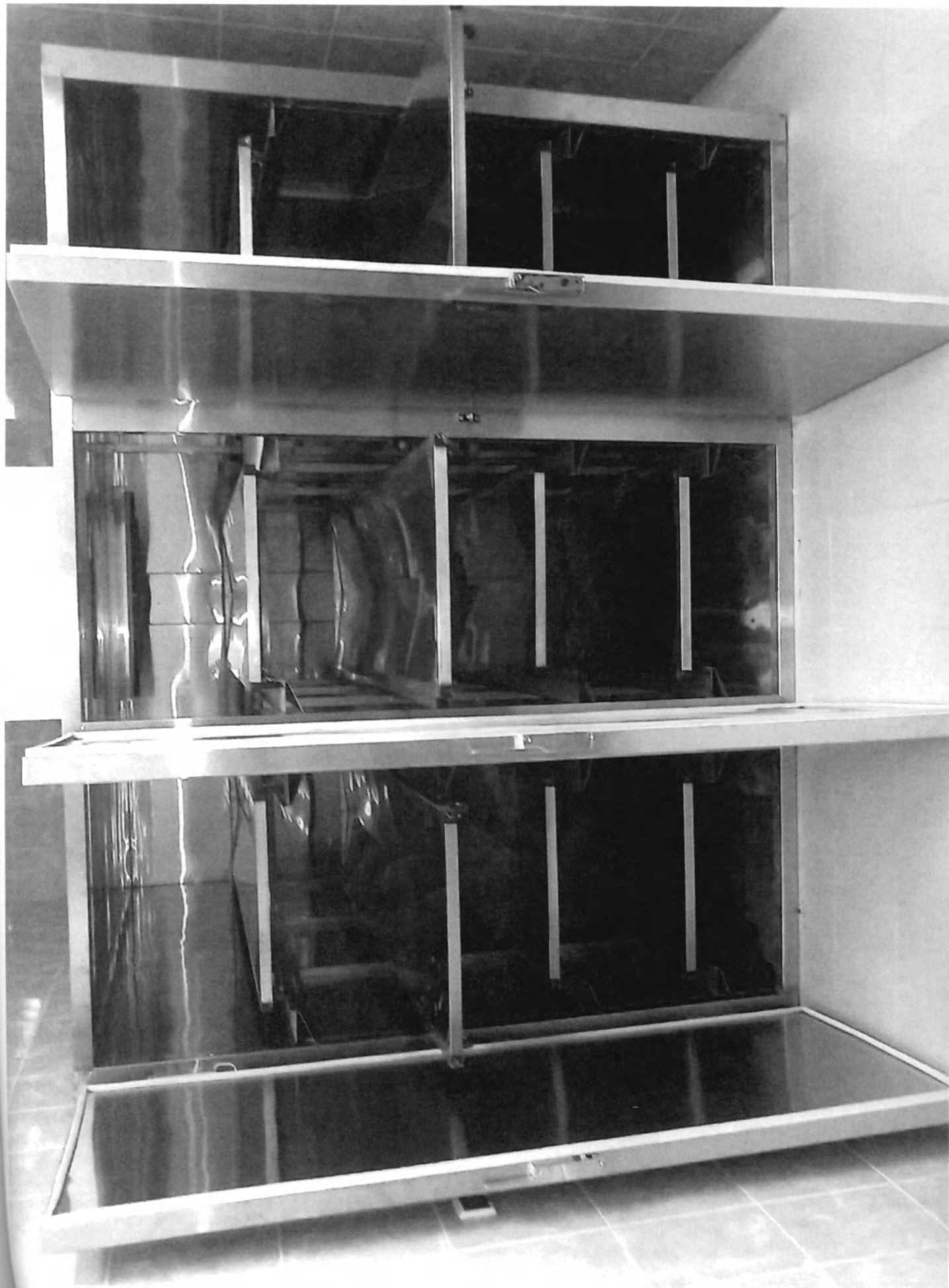
Камера холодильная специальная для хранения тел умерших ЗМУ4-Н, ЗМУ4-К
