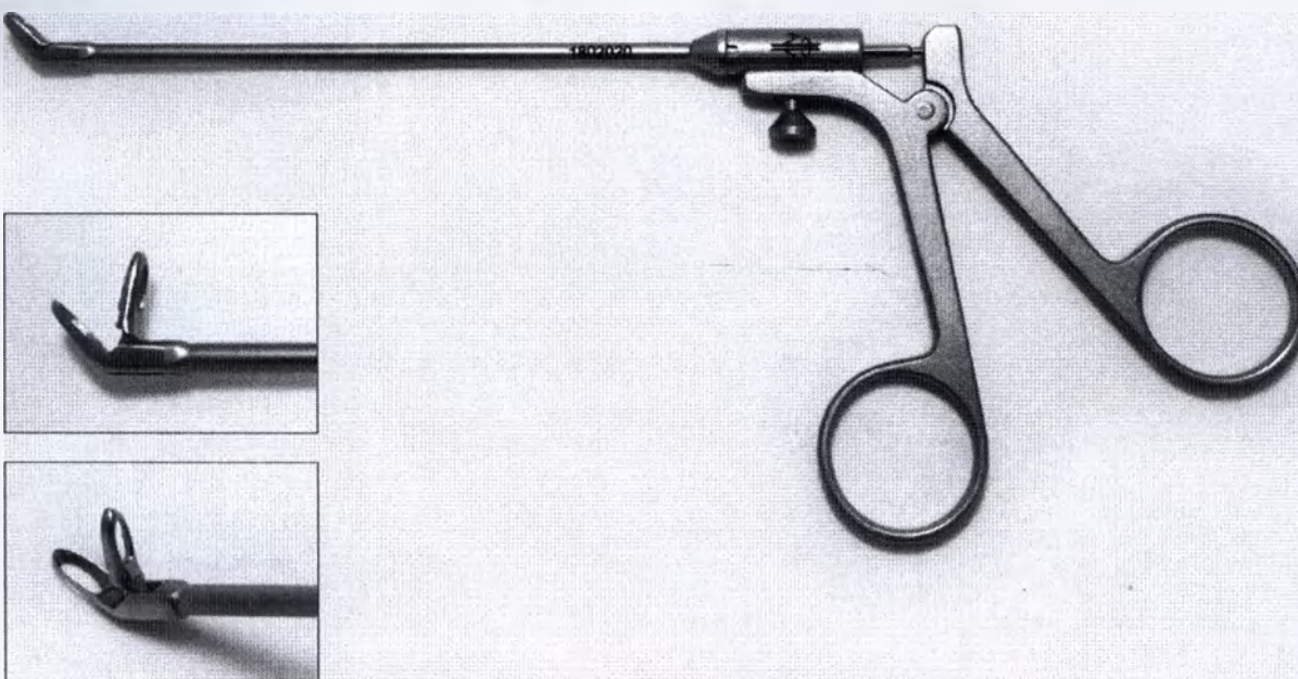
23. Щипцы типа Блексли, бранши повернуты на 45^{\circ} , \varnothing 4 мм
