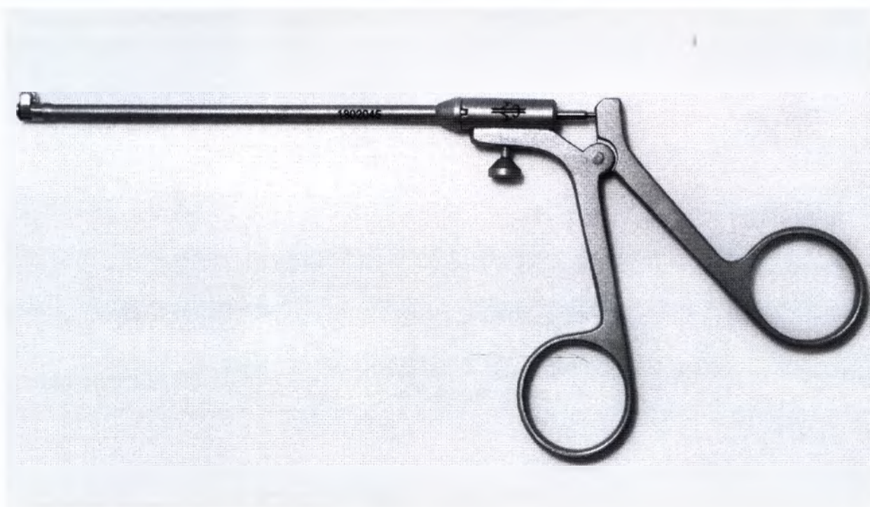
36. Выкусыватель боковой правый
