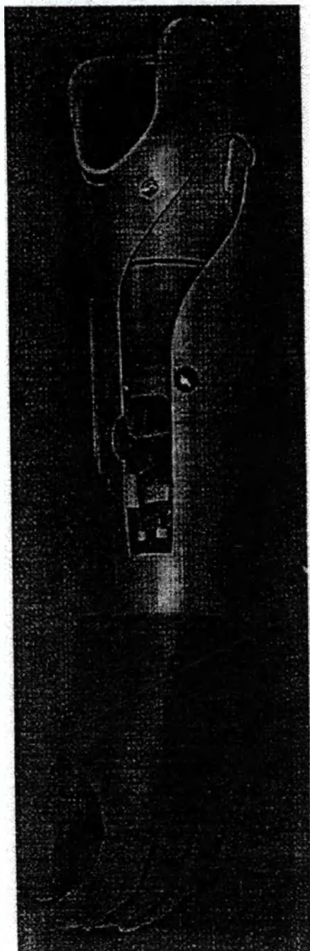
Рисунок А.1 - Протез предплечья с внешним источником энергии фирмы «ОТТО БОКК» ПР2-ВОВ
