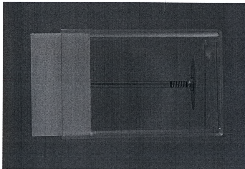
Рис. 19. Диск алмазный дисковидный, с частичным алмазным покрытием нижней стороны рабочей части.
