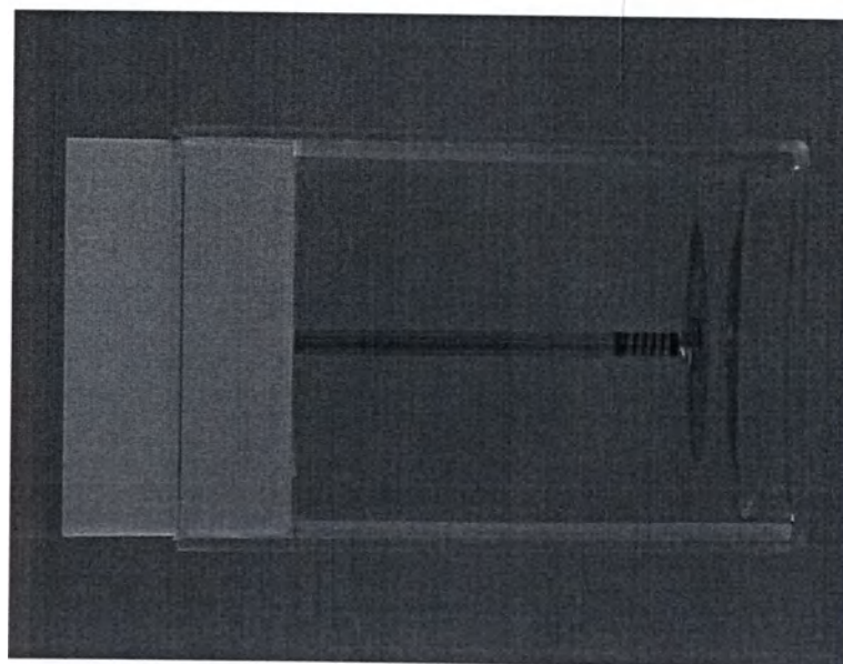
Рис. 15. Диск алмазный дисковидный, с частичным алмазным покрытием рабочей части с обеих сторон.
