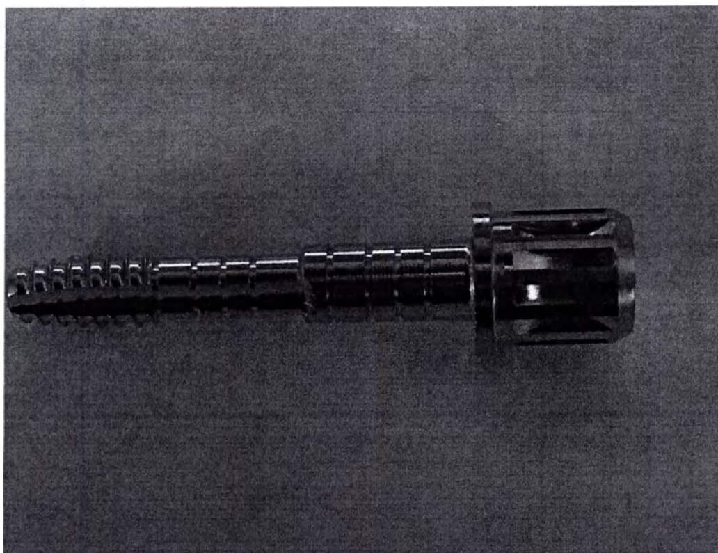
МЕТЧИК Длинный, Ø платформы 4 мм (MASCHIATORE GUIDATO) (PFONG-AT3011)
