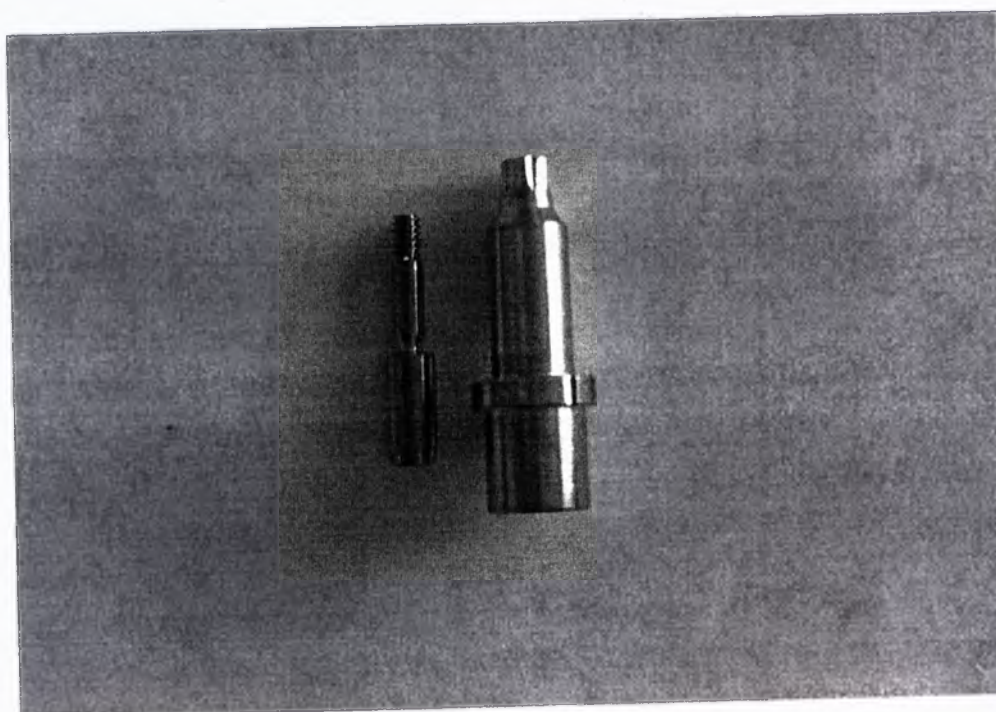
Инструмент направляющий для хирургических шаблонов с винтом, Ø платформы 3.5/4 мм (MONTATORE X GUIDATA + Vite) (PFONG-ATE050)
