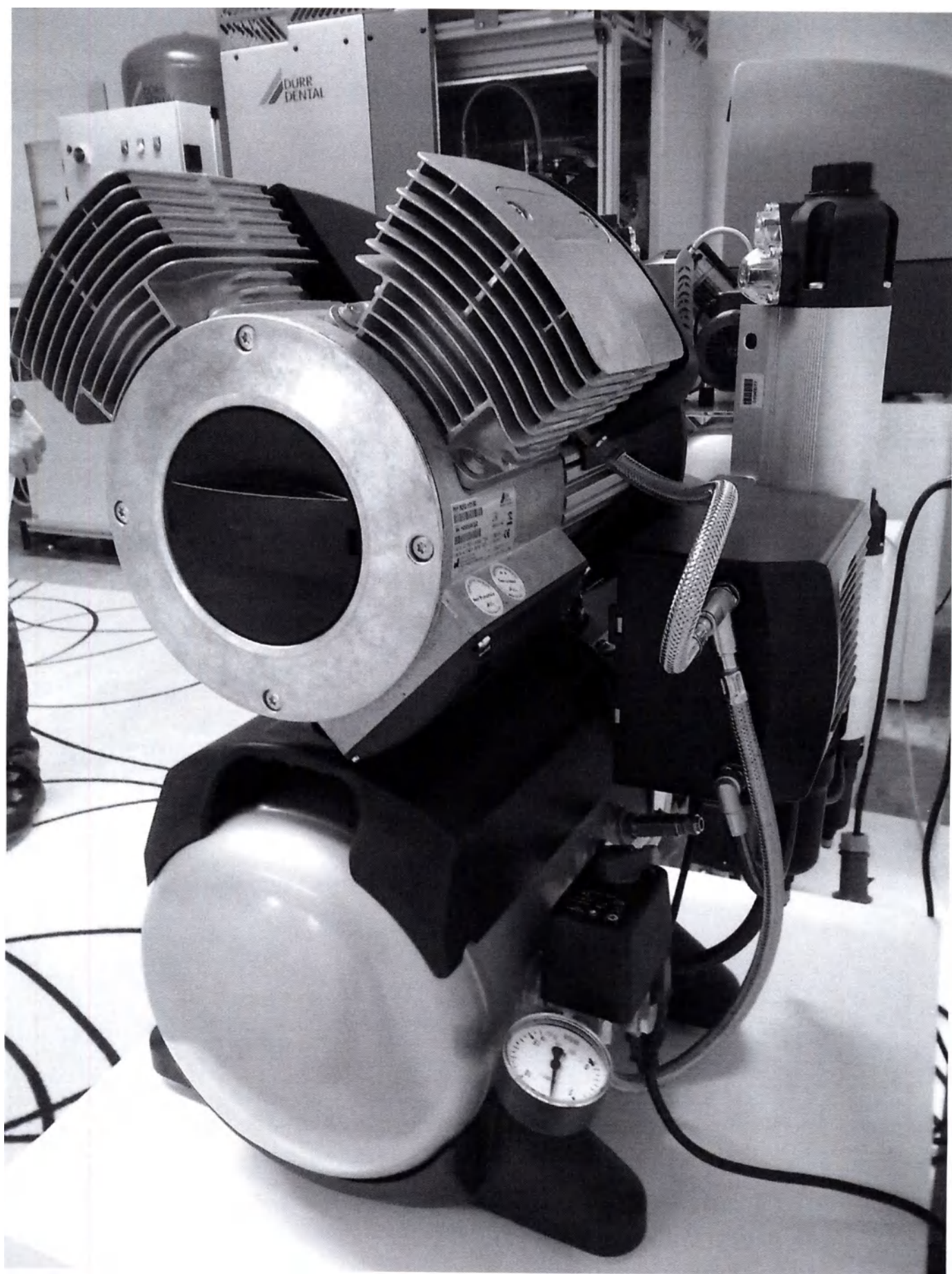
Компрессор стоматологический Tornado 2 с мембранным осушителем
