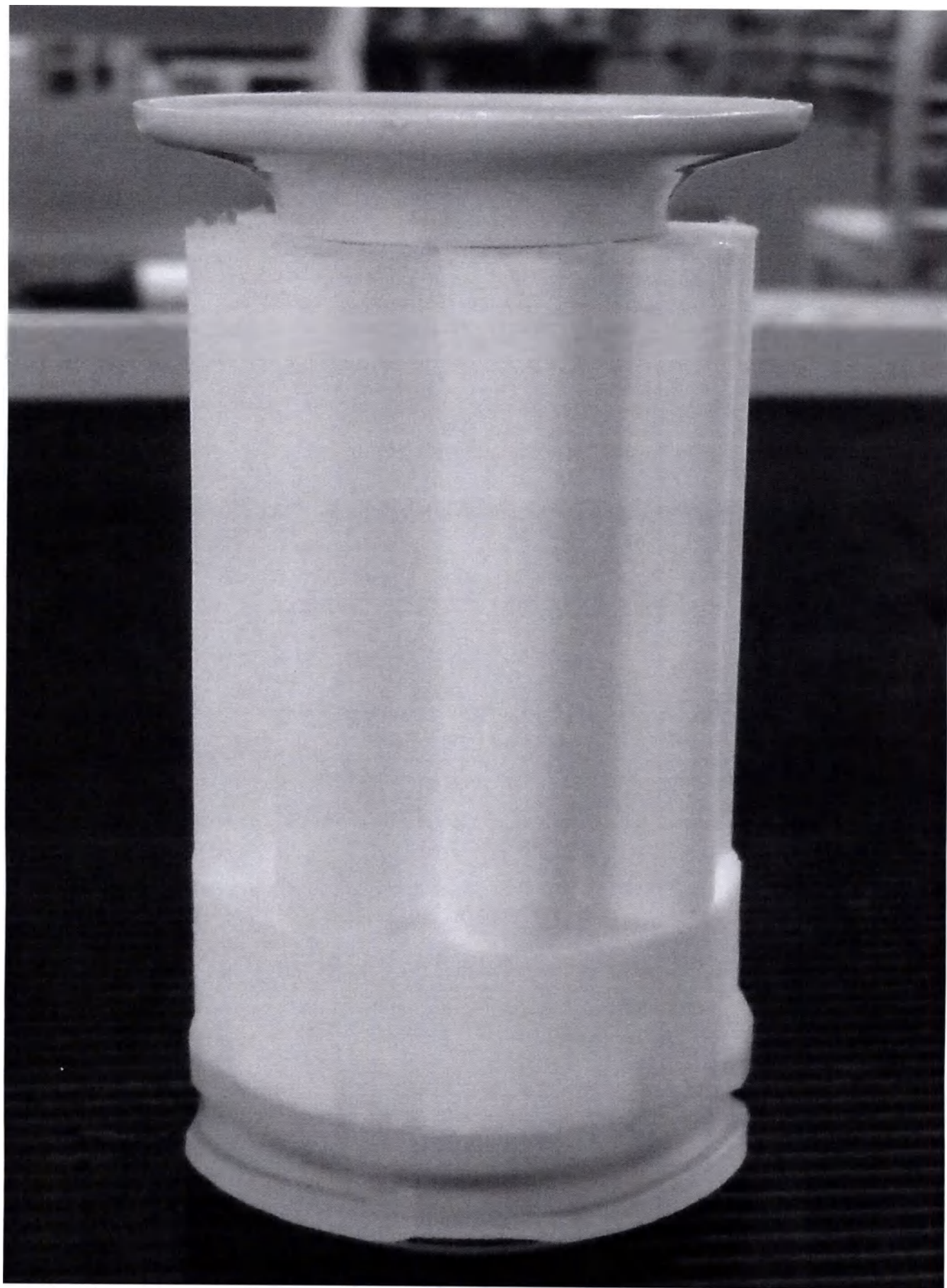
Спечённый фильтр для мембранного осушителя
