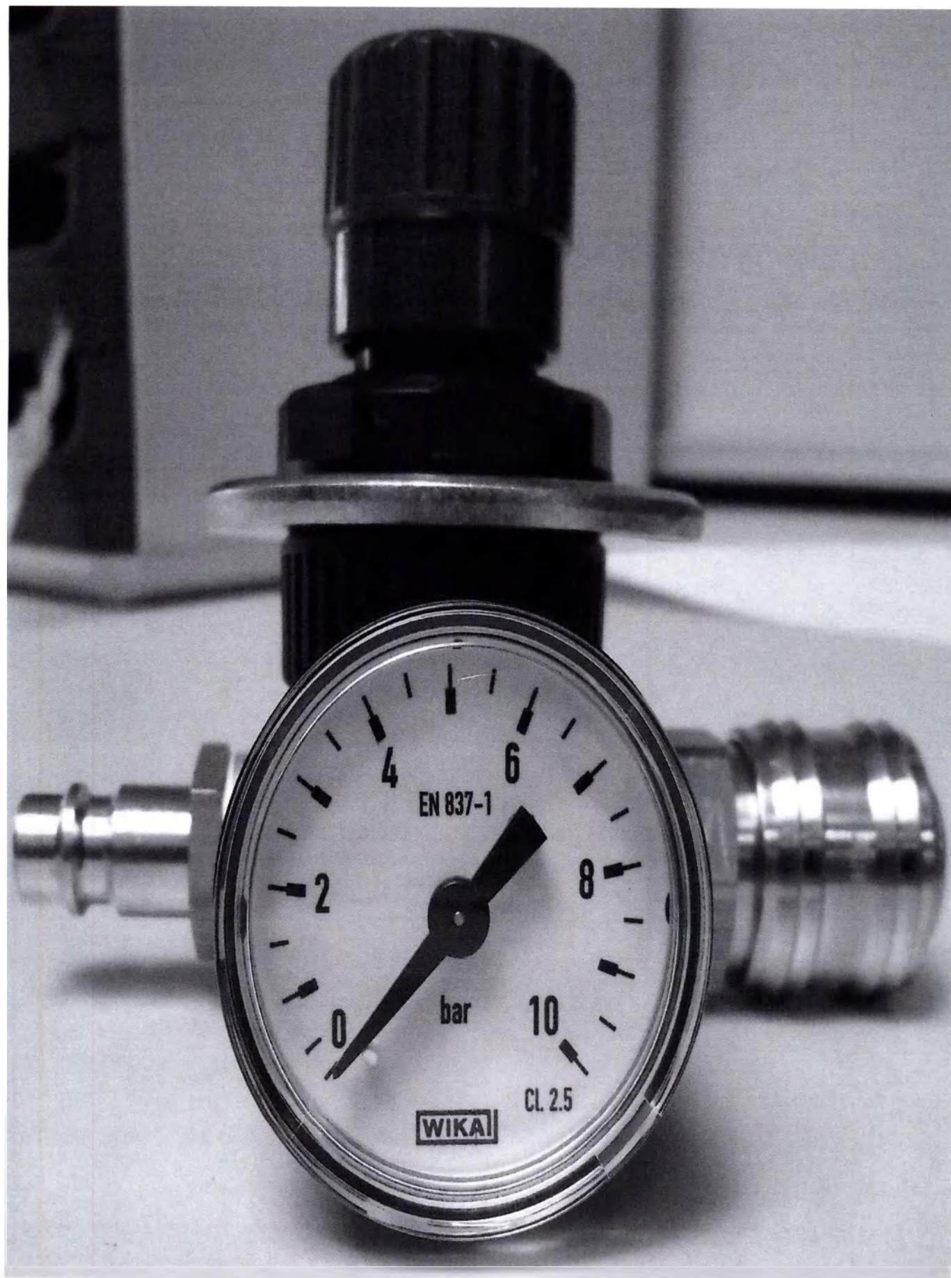
Редукционный клапан
