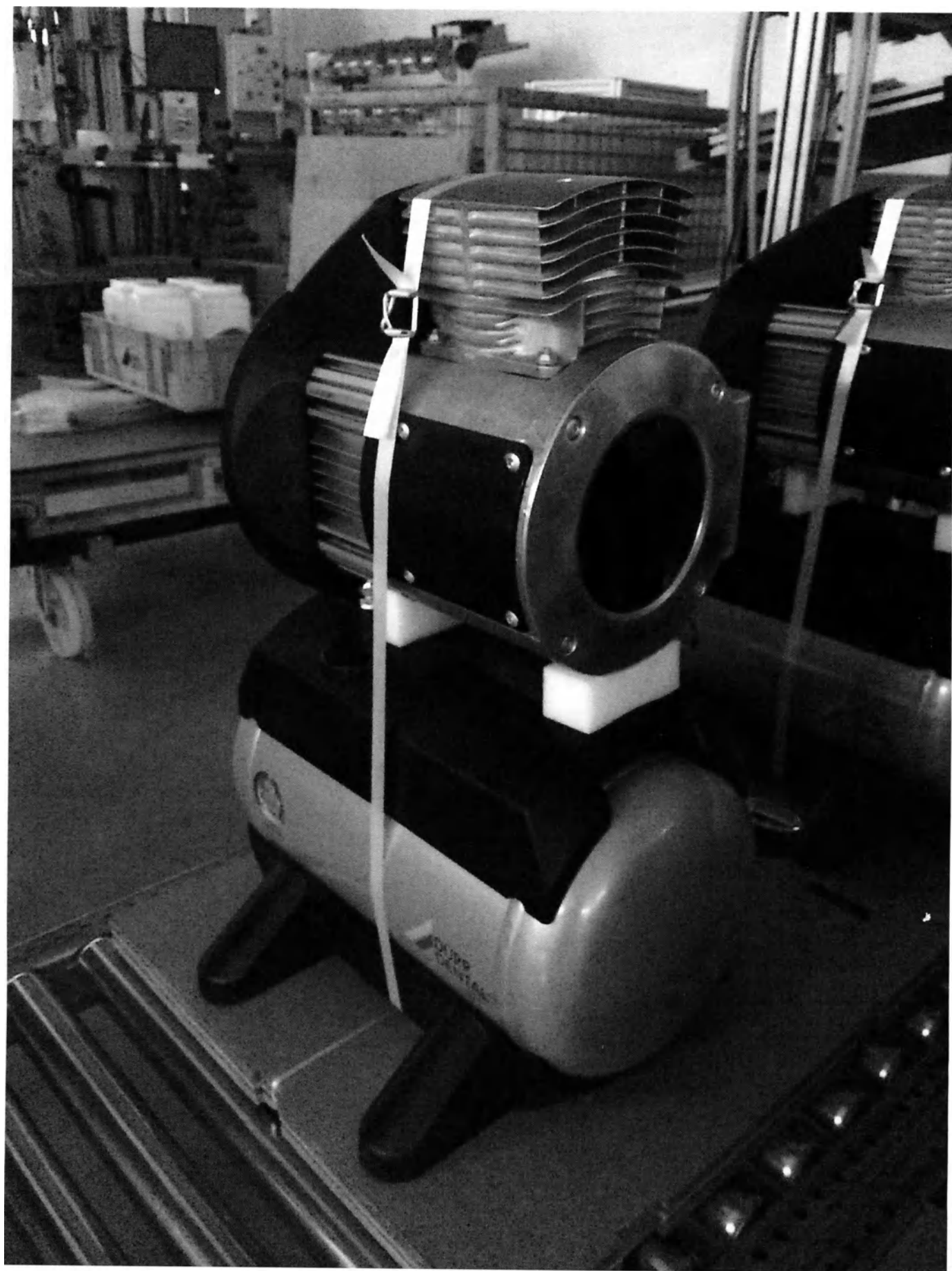
Компрессор стоматологический Tornado 1
