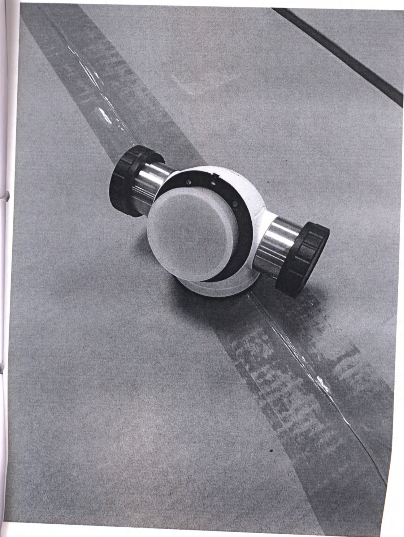
Наклонный двойной светоделитель 80:20
