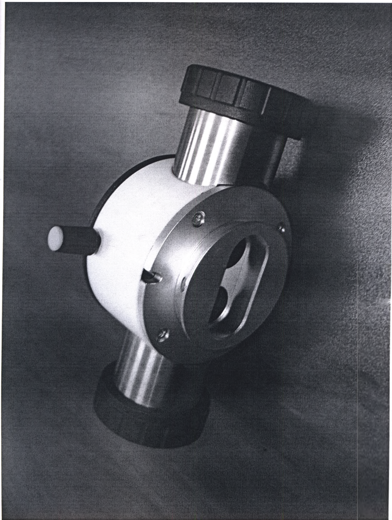
Двойной светоделитель 50:50
