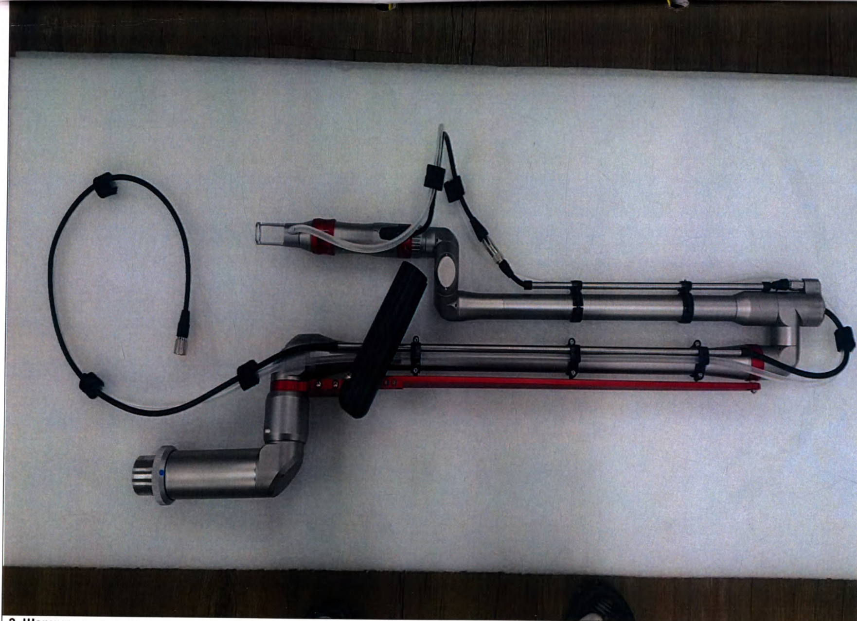
2. Шарнирная консоль.
