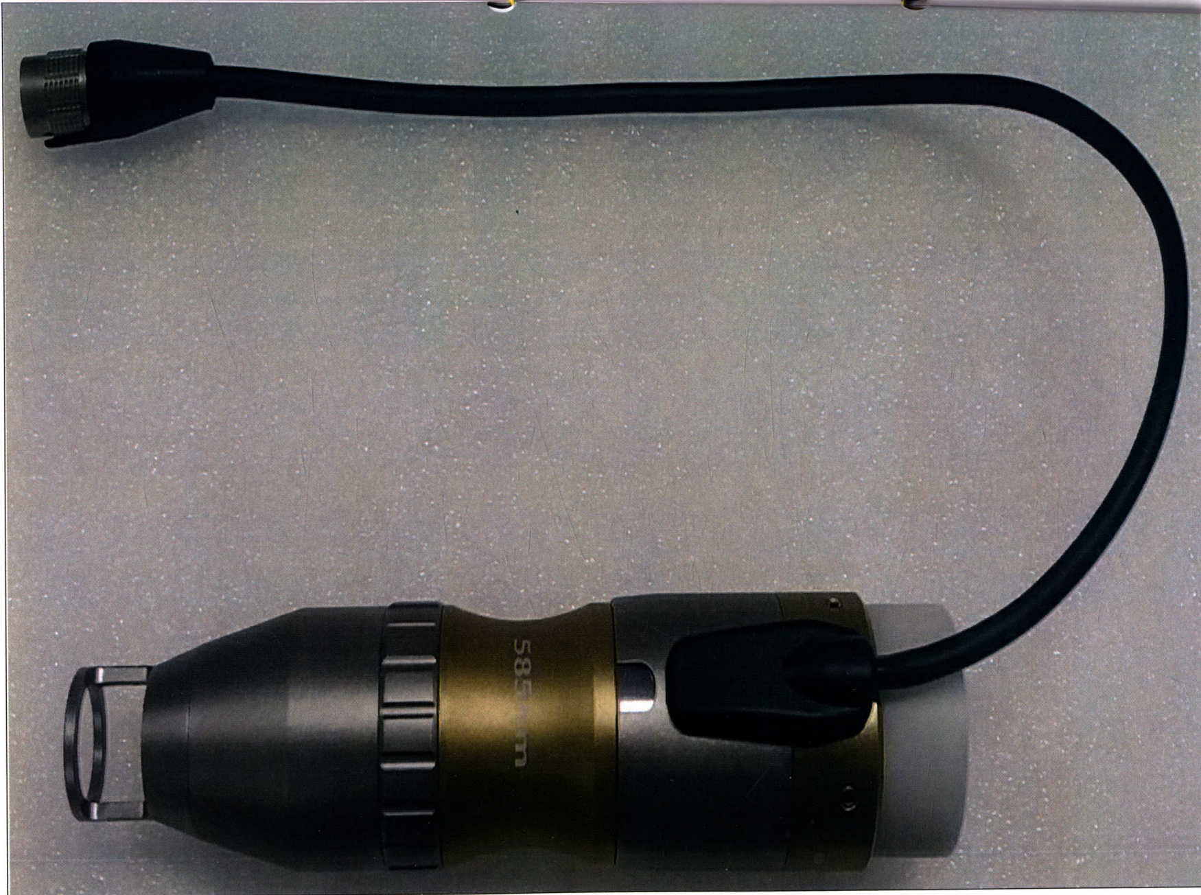
11. Наконечник – рукоятка 585.
