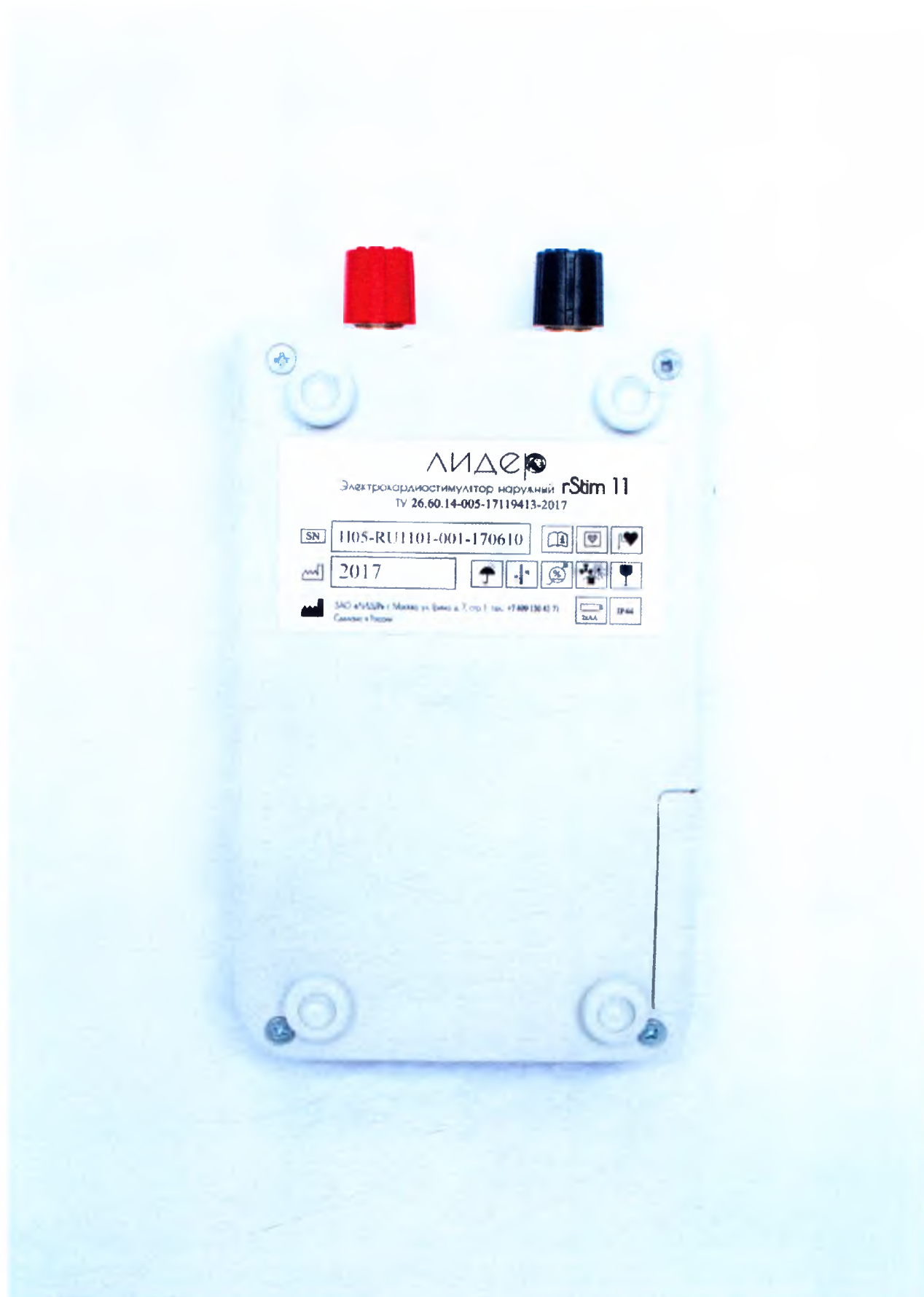
Электрокардиостимулятор наружный однокамерный rStim 11 (вид сзади, маркировка)
