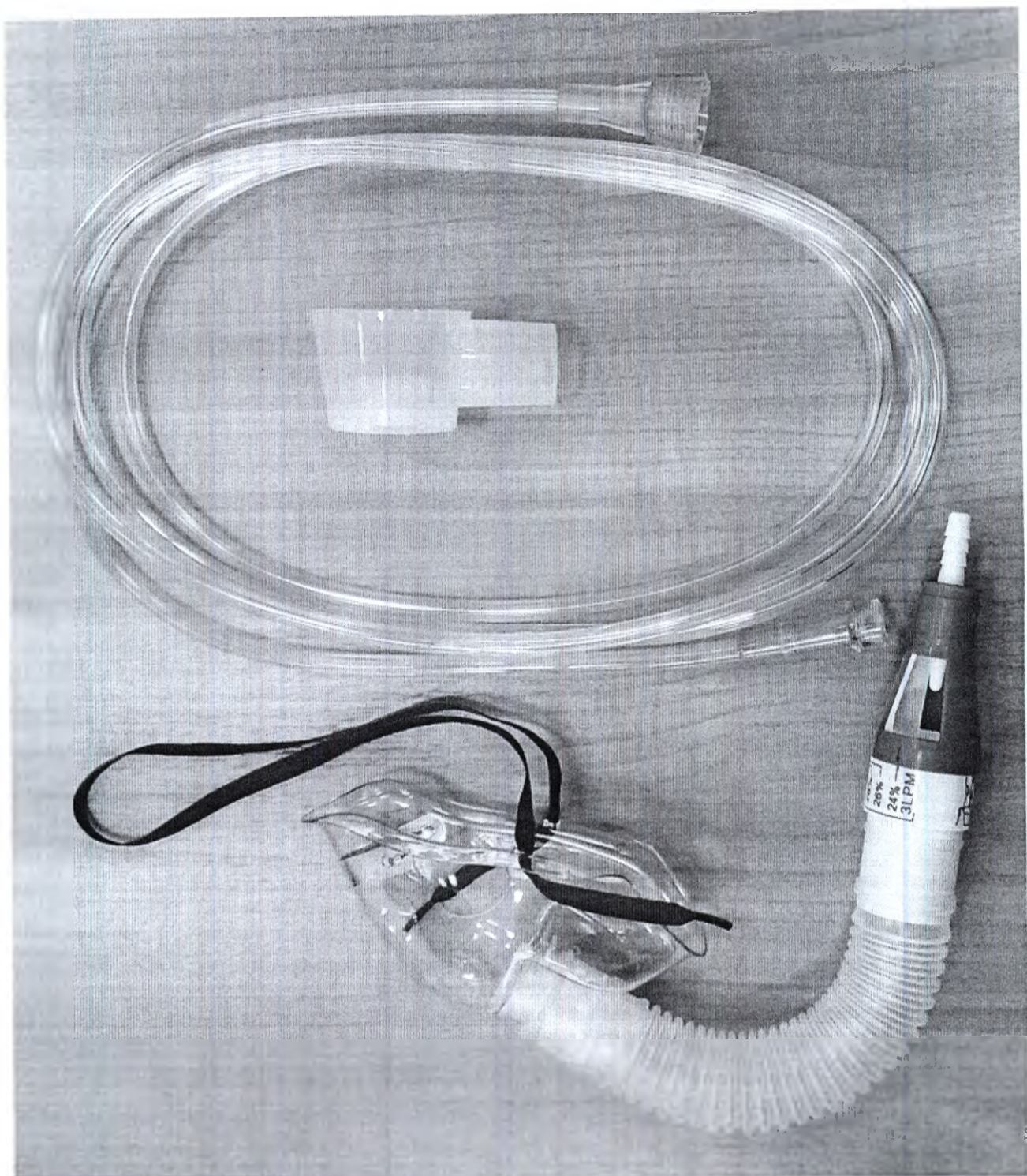
Рисунок 10 – Маска Вентури с регулируемым клапаном Вентури (дилутером) на примере артикула 93-120АММ
