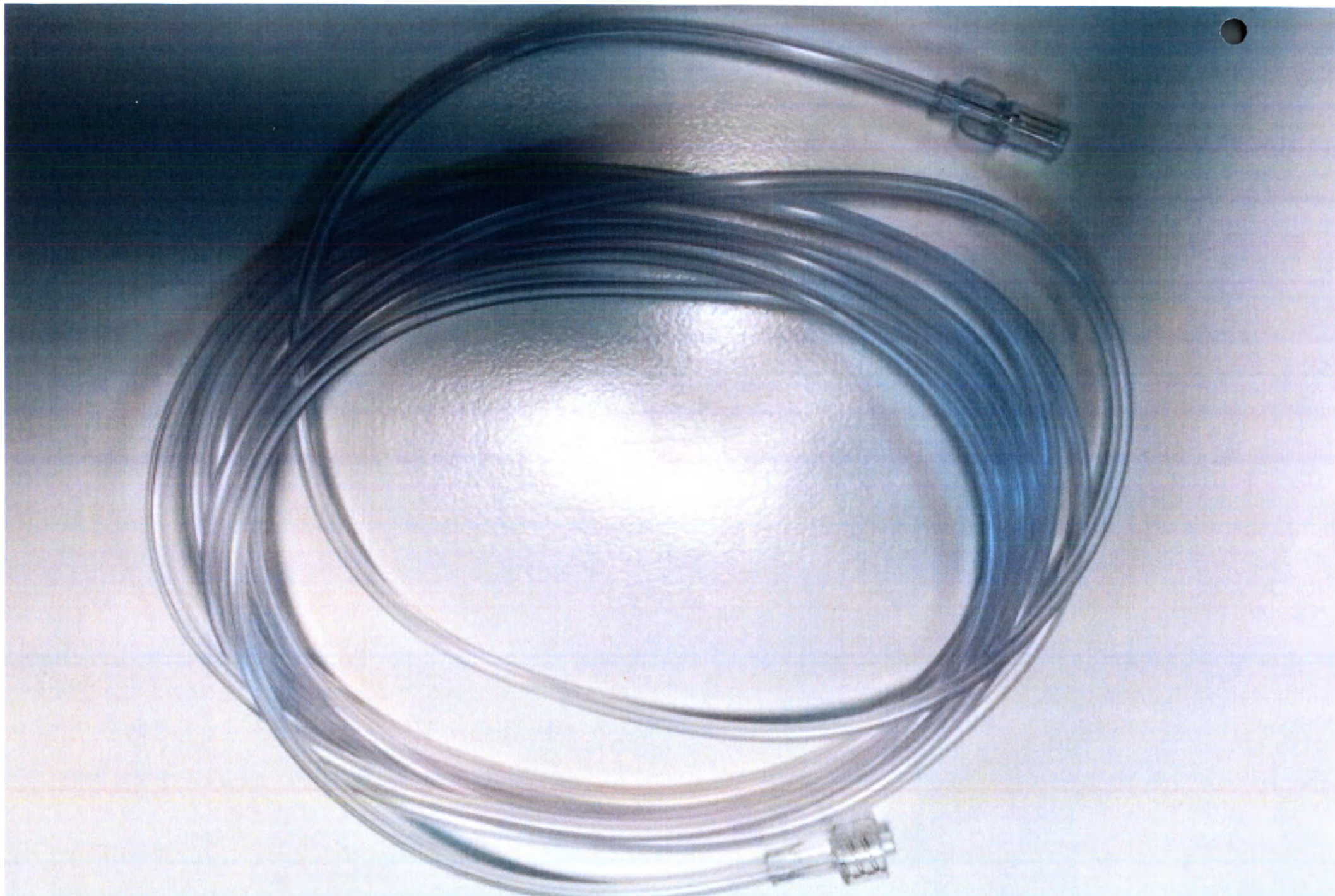
Трубка для отбора проб газа с коннектором типа Луер Мэйл (Luer Male)/Луер Фемэйл (Luer Female), внутренний диаметр 1.27 мм, внешний диаметр 3.33 мм, длиной 3 м
