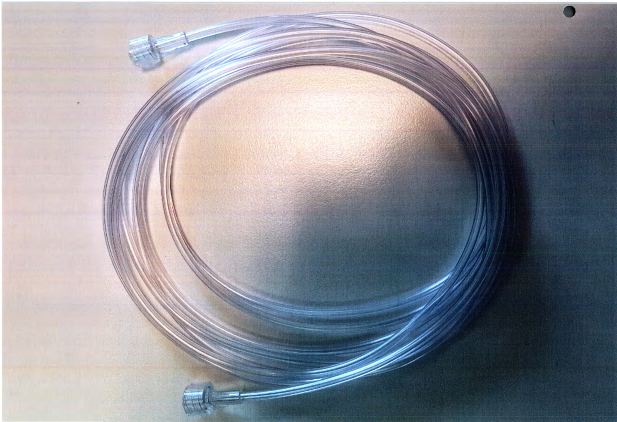
Трубка для отбора проб газа с коннектором типа Луер Мэйл (Luer Male)/Луер Мэйл (Luer Male), внутренний диаметр 1.27 мм, внешний диаметр 3.33 мм длиной 3 м
