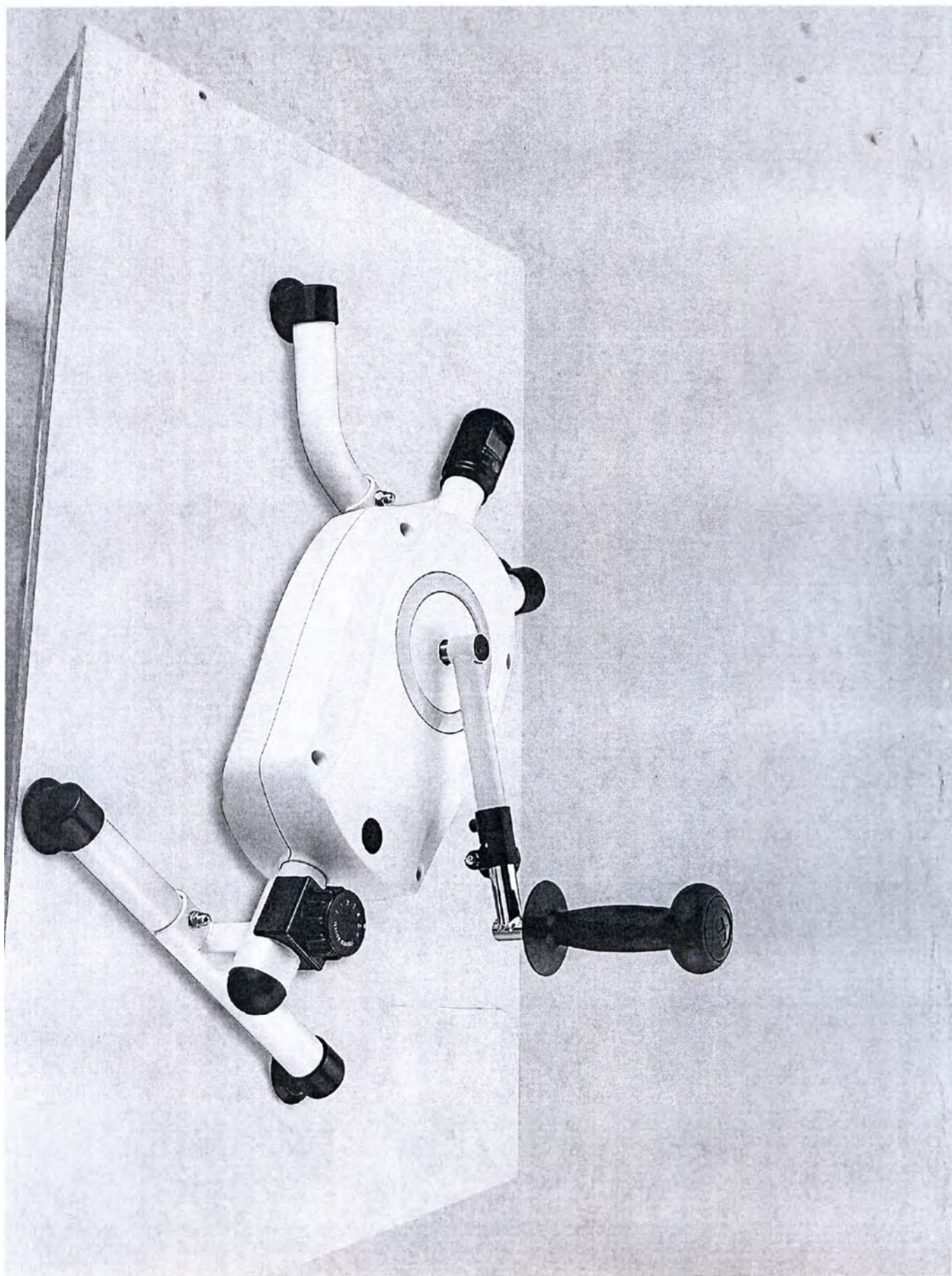
Тренажер для плеча и локтя портативный ЗМ-661С
