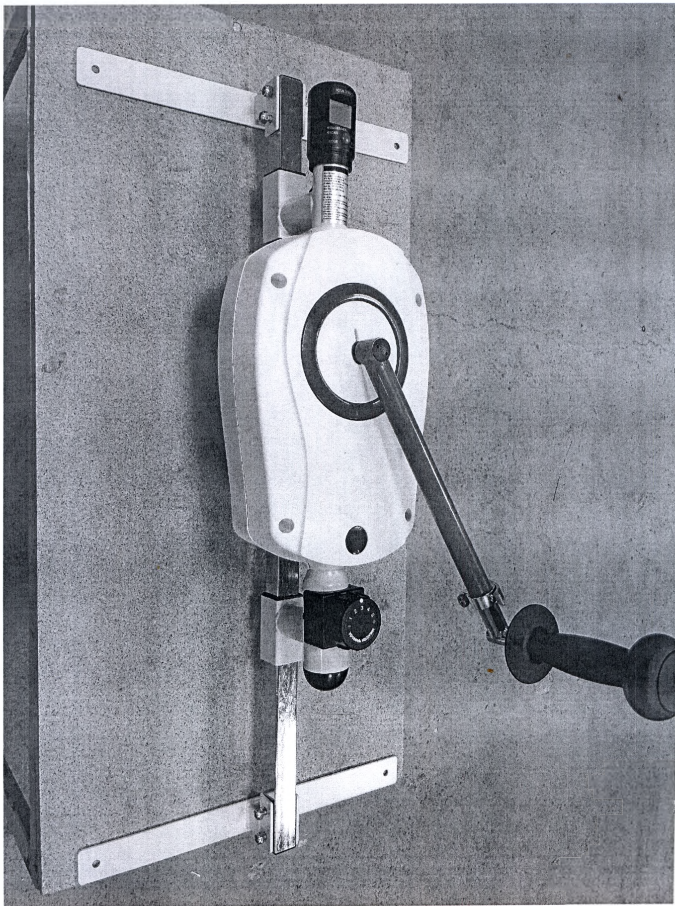
Тренажер для плеча и локтя 3М-660С
