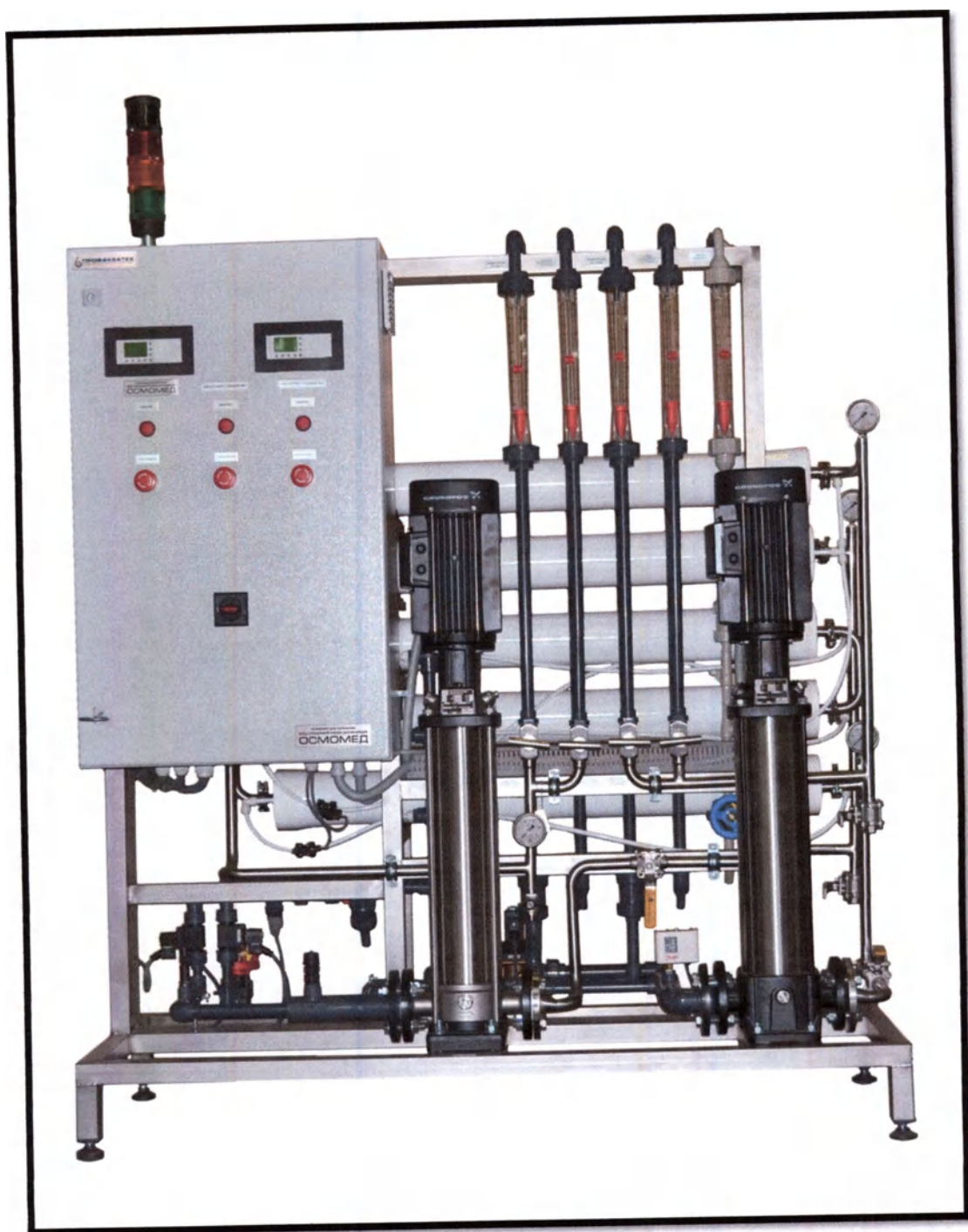
Установка для получения воды очищенной и воды для инъекций ОСМОМЕД-40-3-2 по ТУ 9452-004-20763906-2016
