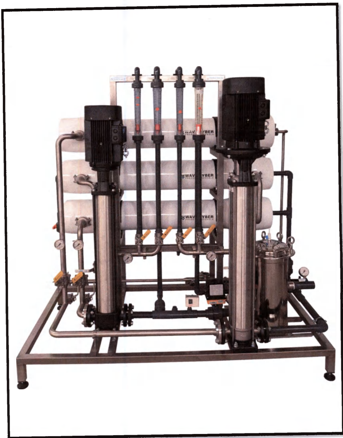
Установка для получения воды очищенной и воды для инъекций ОСМОМЕД 80-2-1 по ТУ 9452-004-20763906-2016
