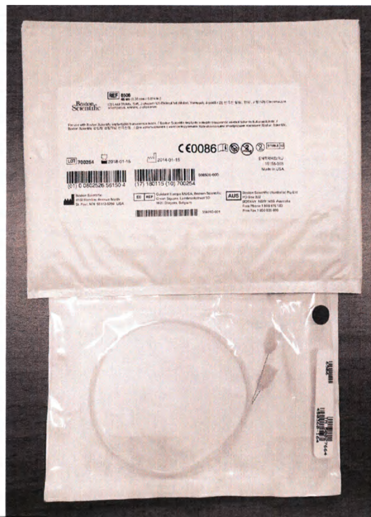
Стилет: Общий вид (49 см)
