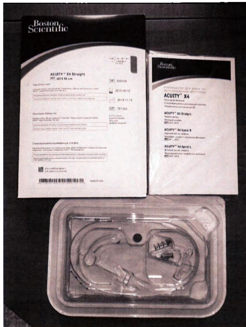
Общий вид (модель: 4672)
