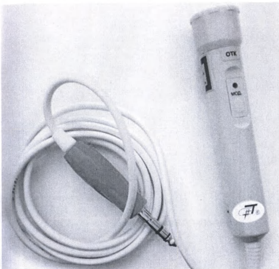
Лазерная излучающая головка КЛО-530-50
