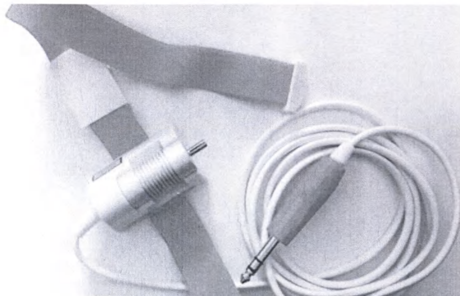
Лазерная излучающая головка КЛ-ВЛОК-808-40
