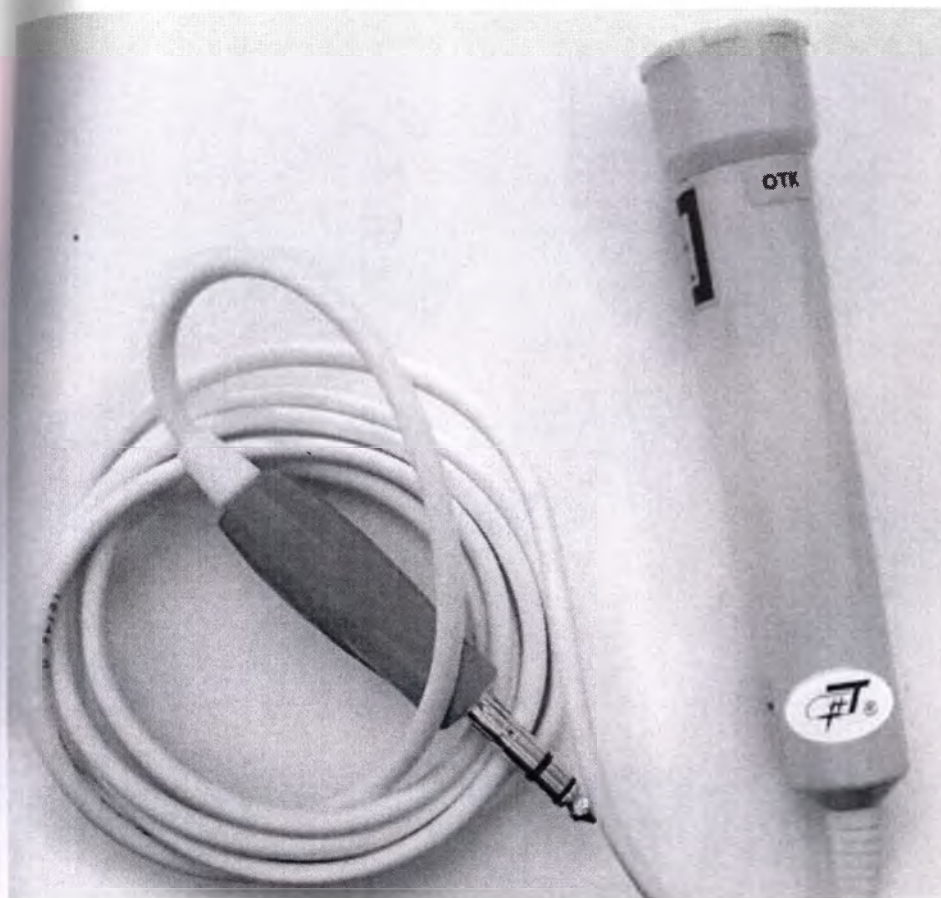
Лазерная головка импульсного излучения ЛО2
