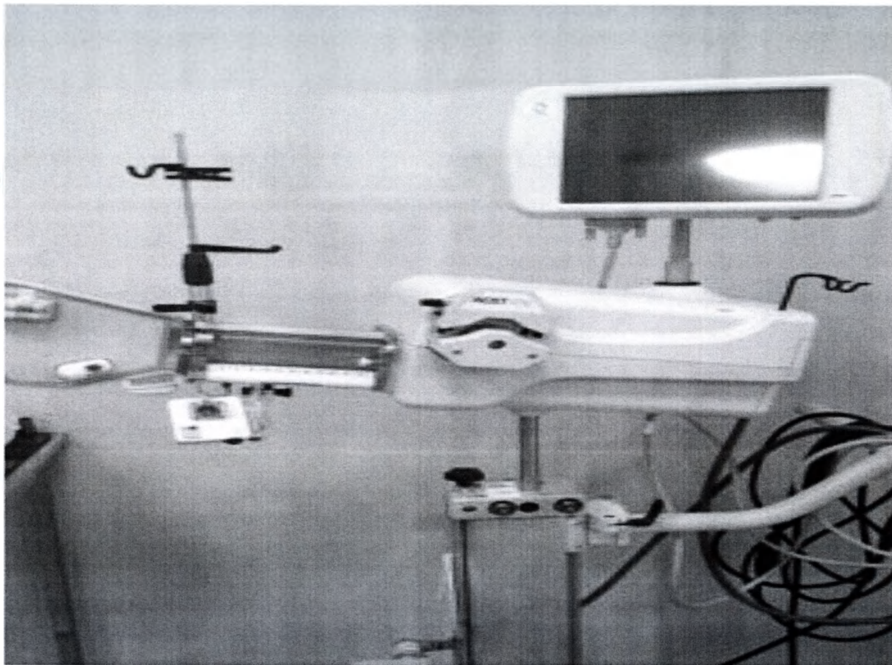
Устройство автоматическое для введения контрастного вещества.
