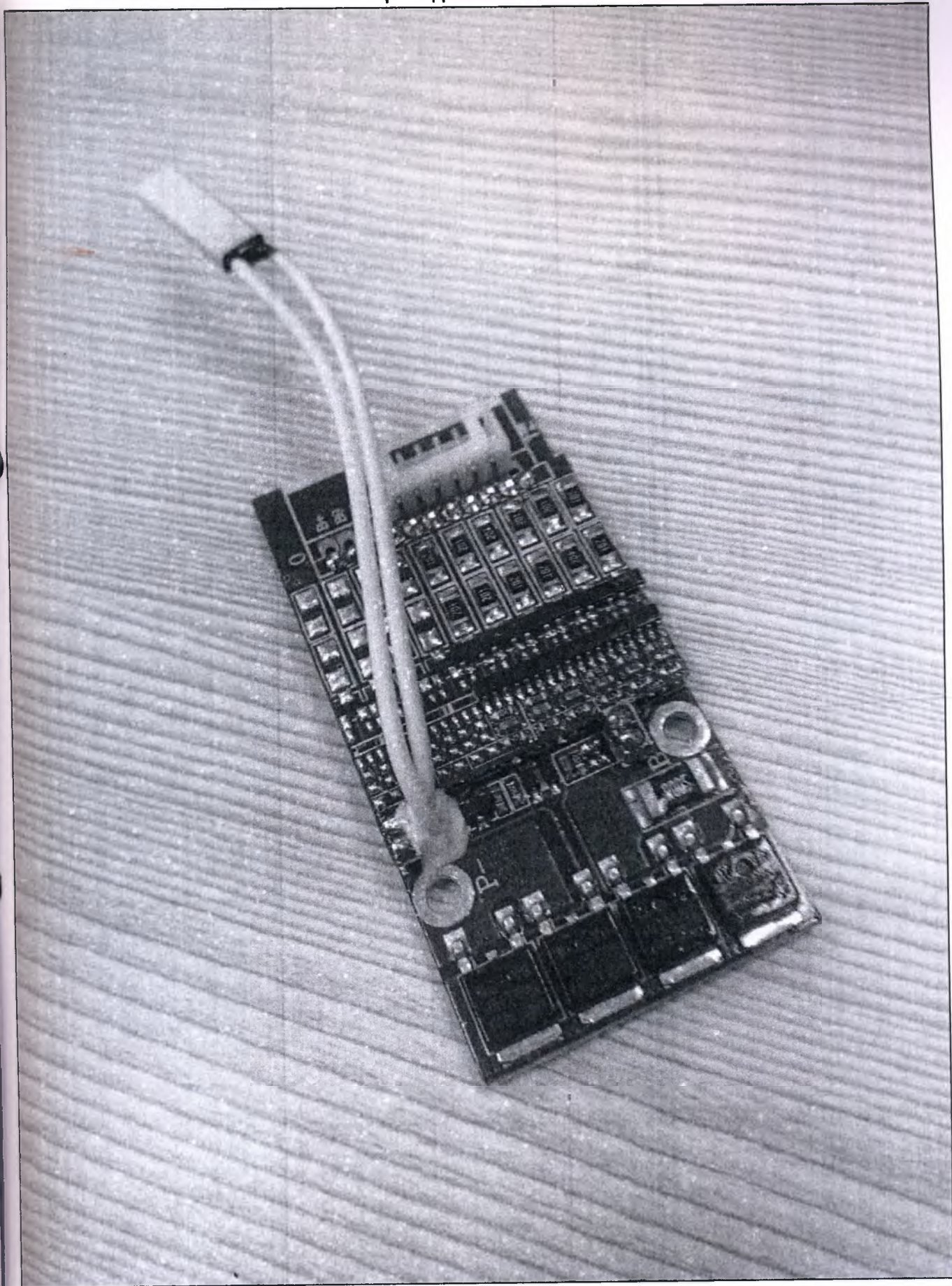
Контроллер заряда/разряда аккумулятора
