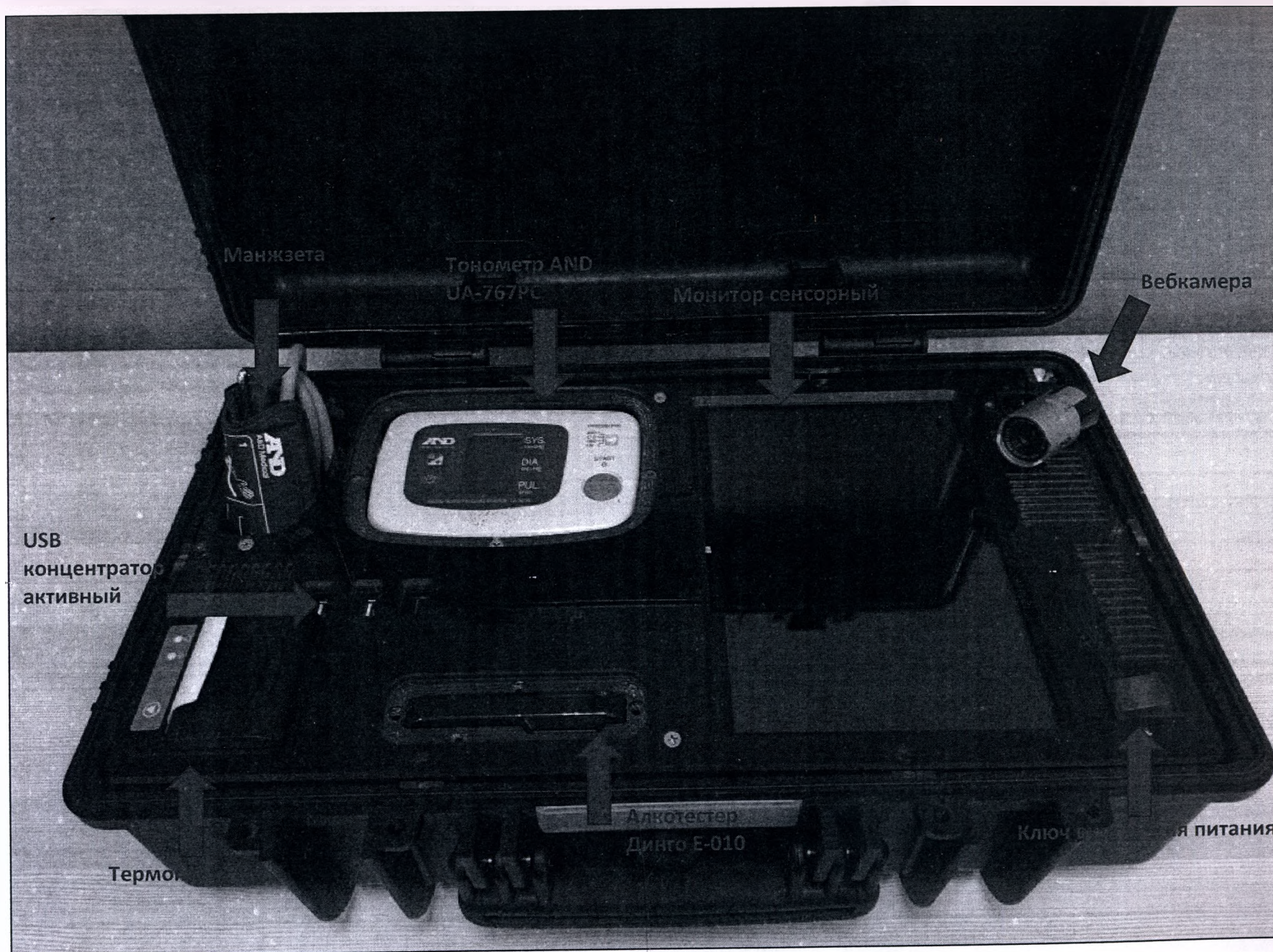
Вид спереди со снятыми крышками алкотестера и тонометра
