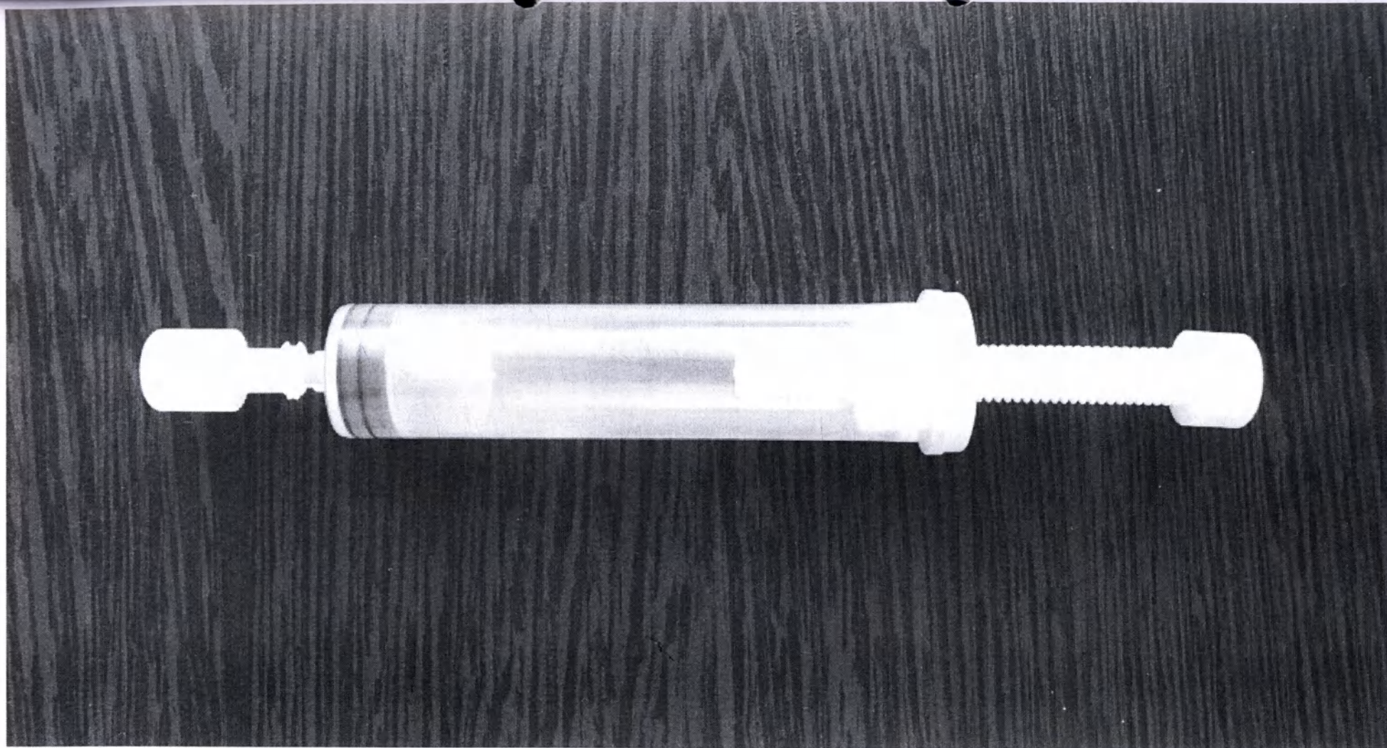
Шприц-пробирка полимерная центрифужная, стерильная CORTEXIL (КОРТЕКСИЛ) по ТУ 32.50.50-001-76853870-2018 объемом 10 мл, с концентрическим расположением наконечника в сборном виде
