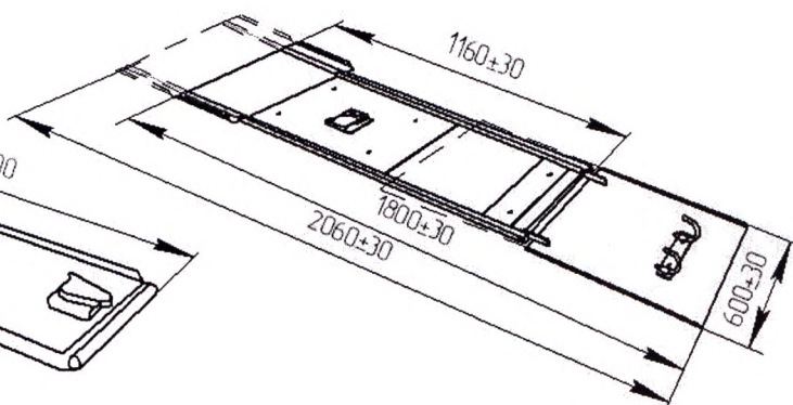
Рисунок В.33. Устройство приемное
