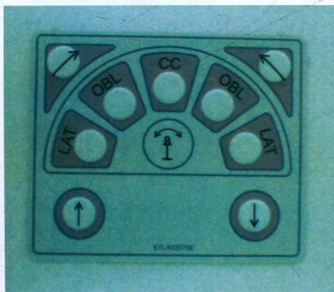
Кнопки управления перемещениями СУ
