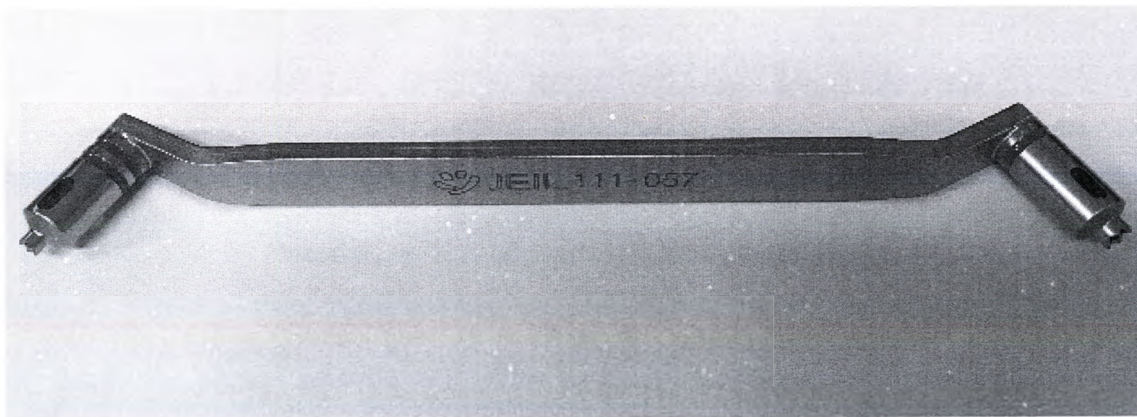
Направитель сверла 111-057
