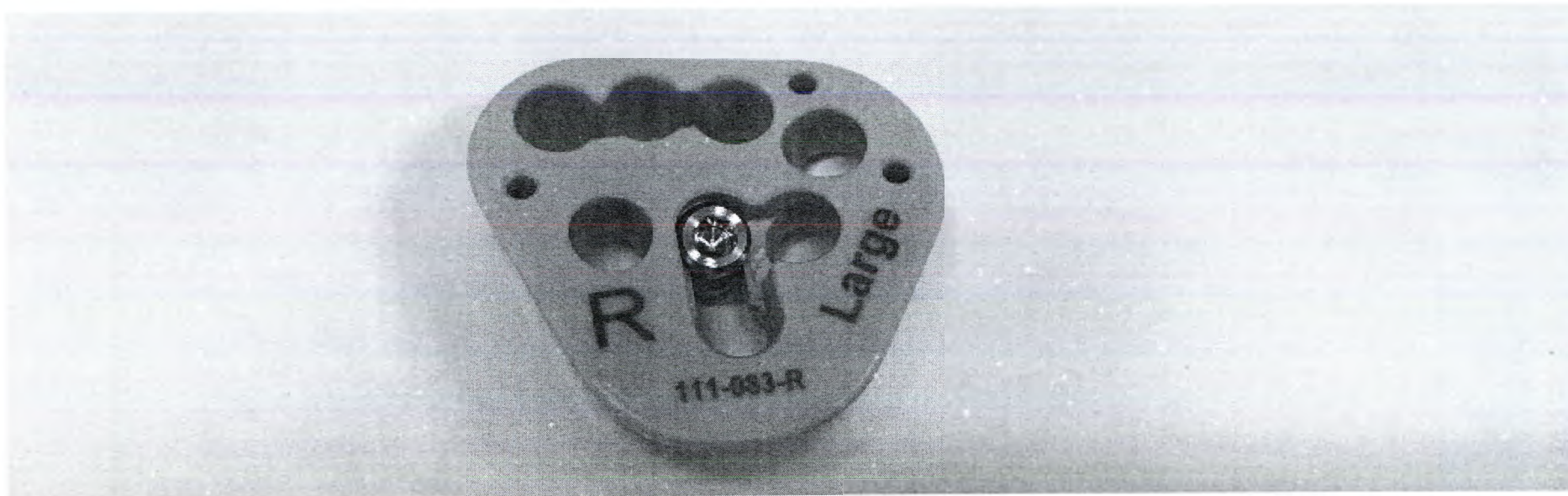
Блокировка направляющего сверла 111-083-R
