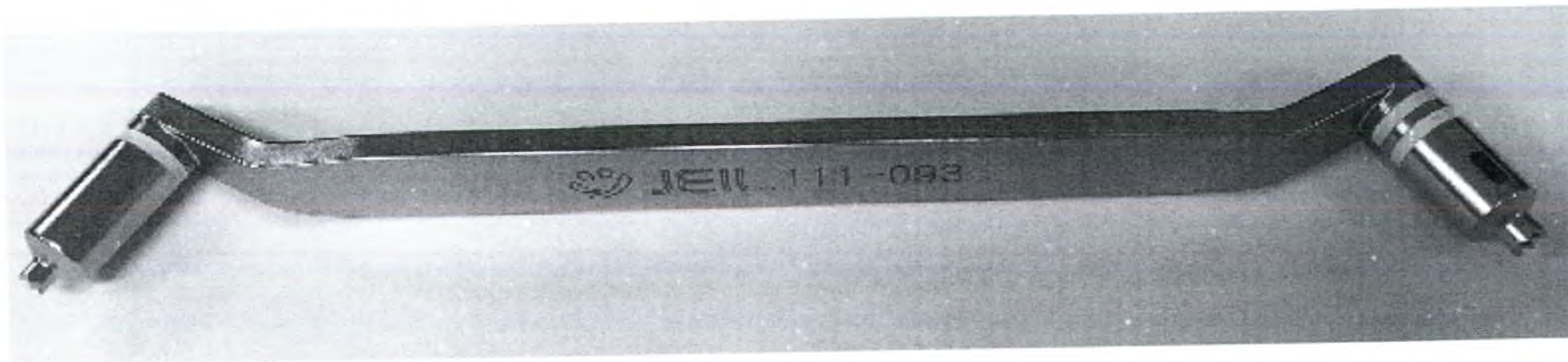
Направитель сверла 111-093
