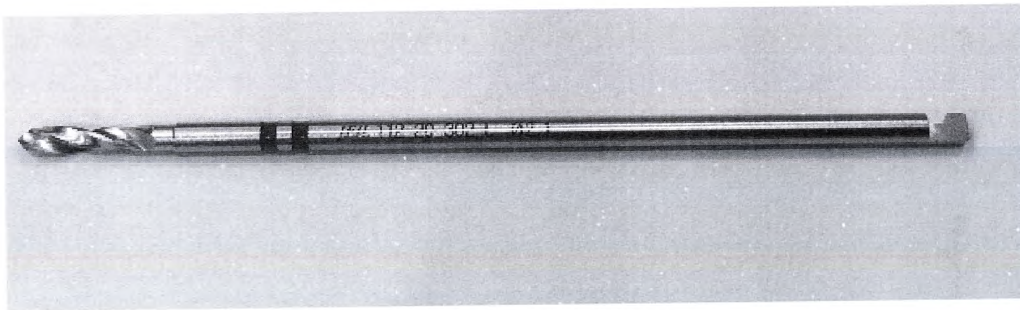
Сверло 112-23-302-L
