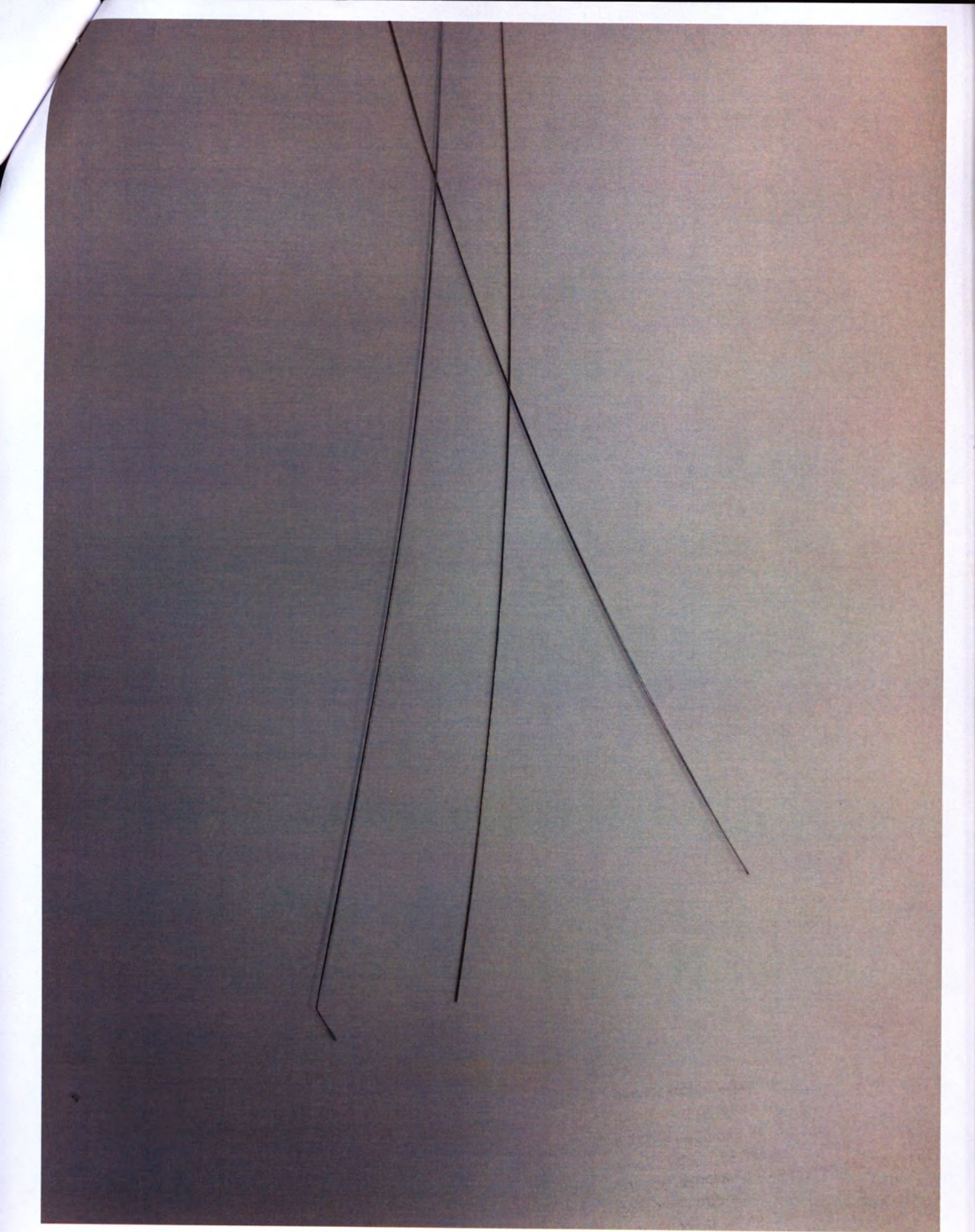
Рис. 4. Проводник внутрисосудистый Synchro. Варианты исполнения: Synchro 2 , длиной 300 см, Synchro-10, длиной 200 см, Synchro-14, длиной 200 см. Без упаковки.
