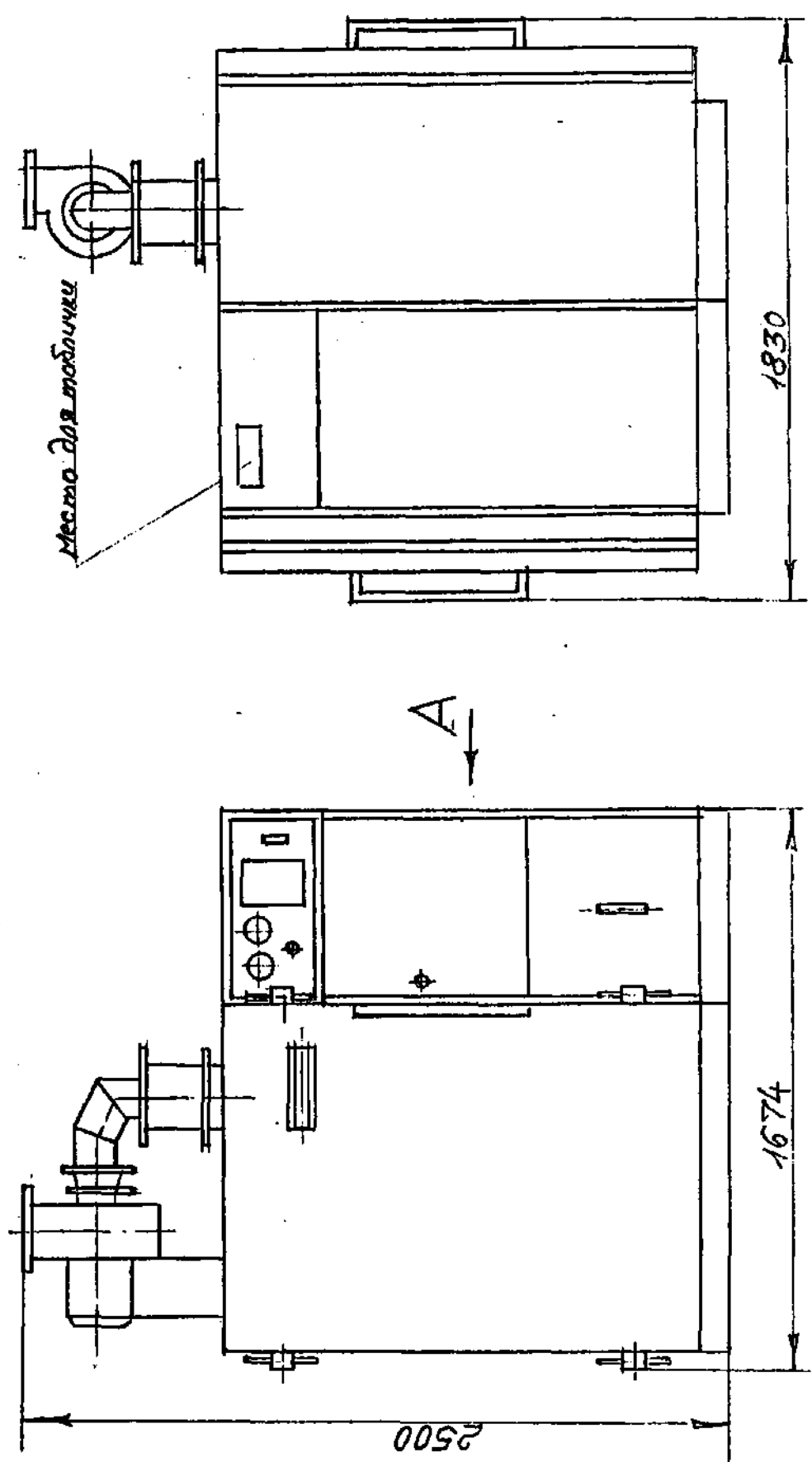
Рис. 1 Камера дезинфекционная ВФС-2/1,4
