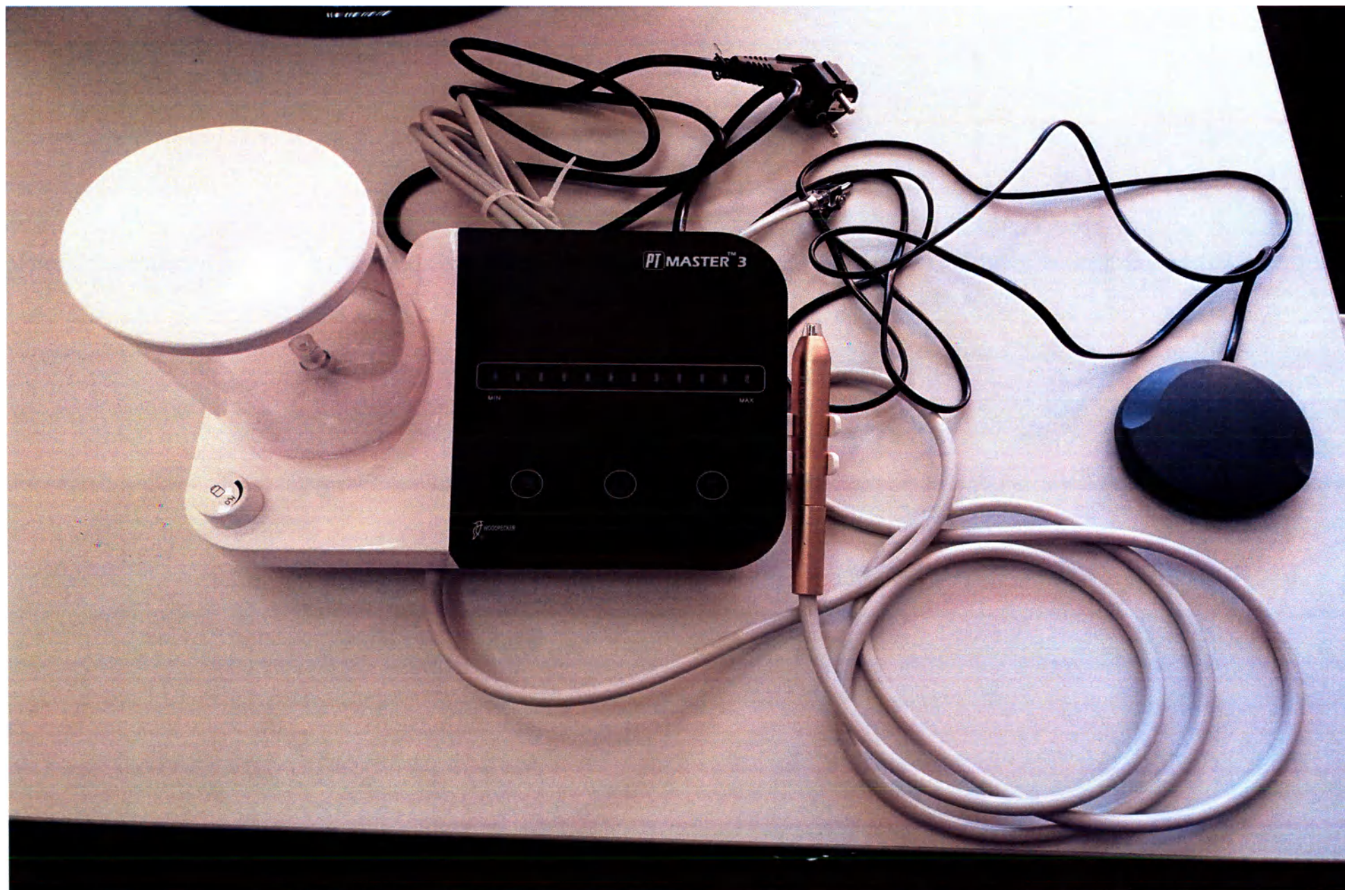
Скейлер ультразвуковой серии DTE, модель: PT3 (общий вид в сборе)
