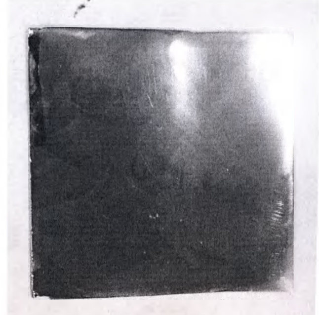
Защитно-упрочняющее покрытие из нитрида циркония на основе из стали марки 12Х18Н9Т
