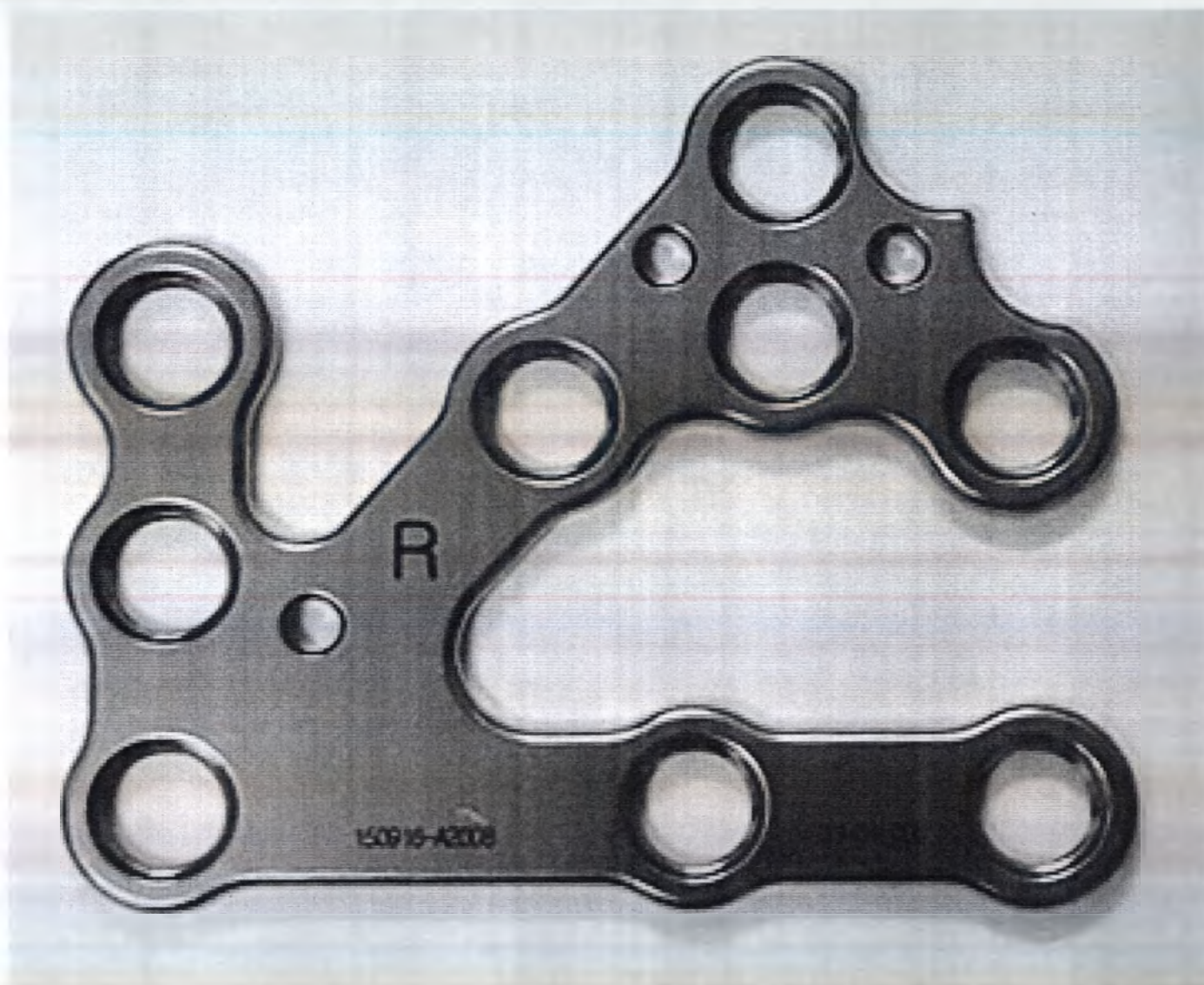
Пластина ARIX Foot System Bone Plate F35-CR-009; Внешний вид моделей F35-CR-009; F35-CL-009 идентичен
