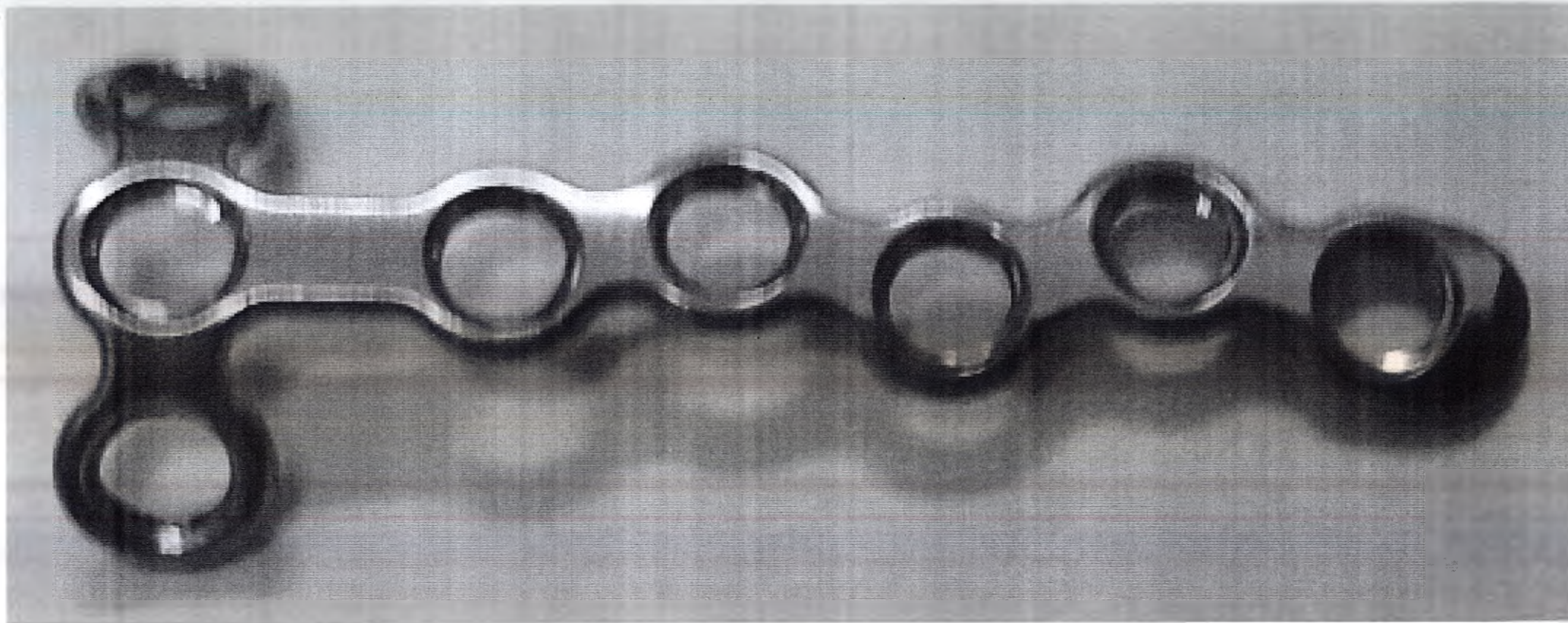
Пластина ARIX Hand System Bone Plate H2L-TP-008;
