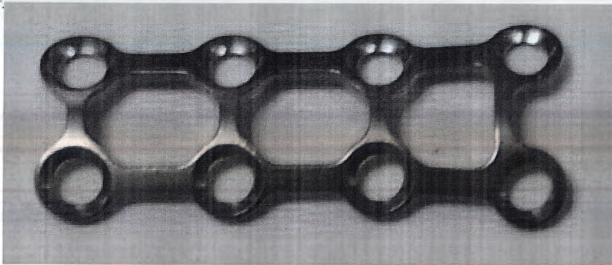
Пластина ARIX Hand System Bone Plate H1-QD-108;
