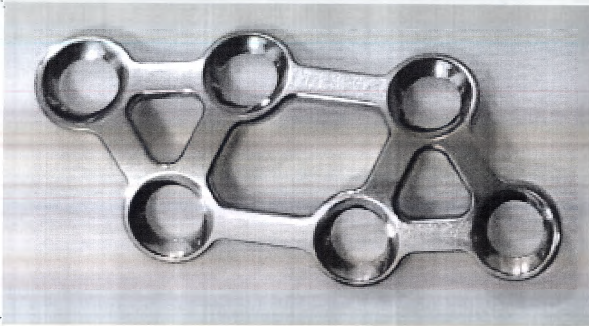
Пластина ARIX Hand System Bone Plate H1-QD-306-R; Внешний вид моделей H1-QD-306-R; H1-QD-306-L идентичен
