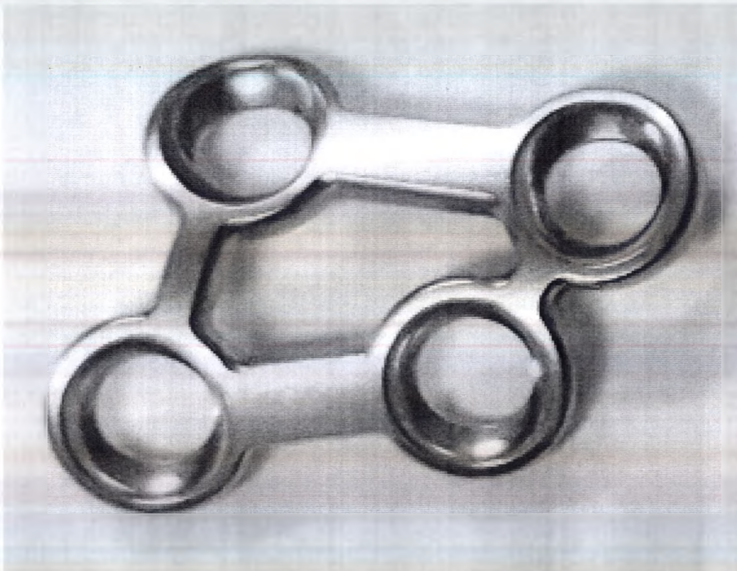
Пластина ARIX Hand System Bone Plate H2-SQ-304-L; Внешний вид моделей H2-SQ-304-L; H2-SQ-304-R идентичен
