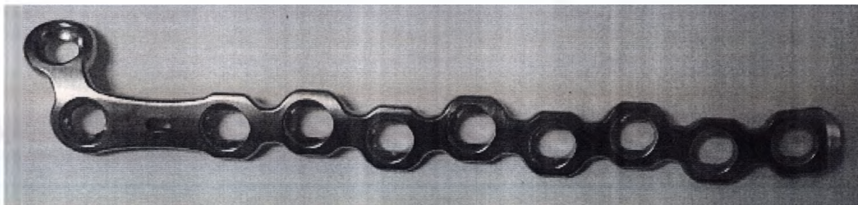
Пластина ARIX Hand System Bone Plate H2-LL-010-CP;
