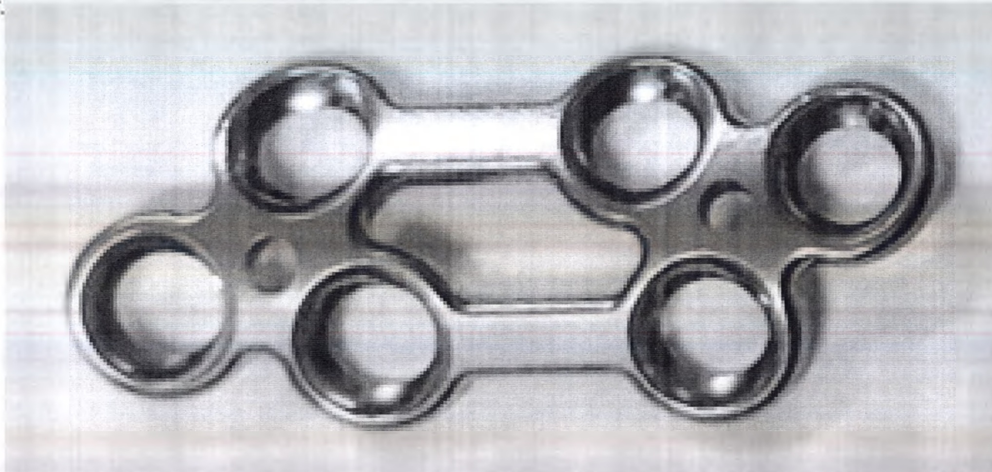
Пластина ARIX Hand System Bone Plate H2-QD-306-L; Внешний вид моделей H2-QD-306-L; H2-QD-306-R идентичен
