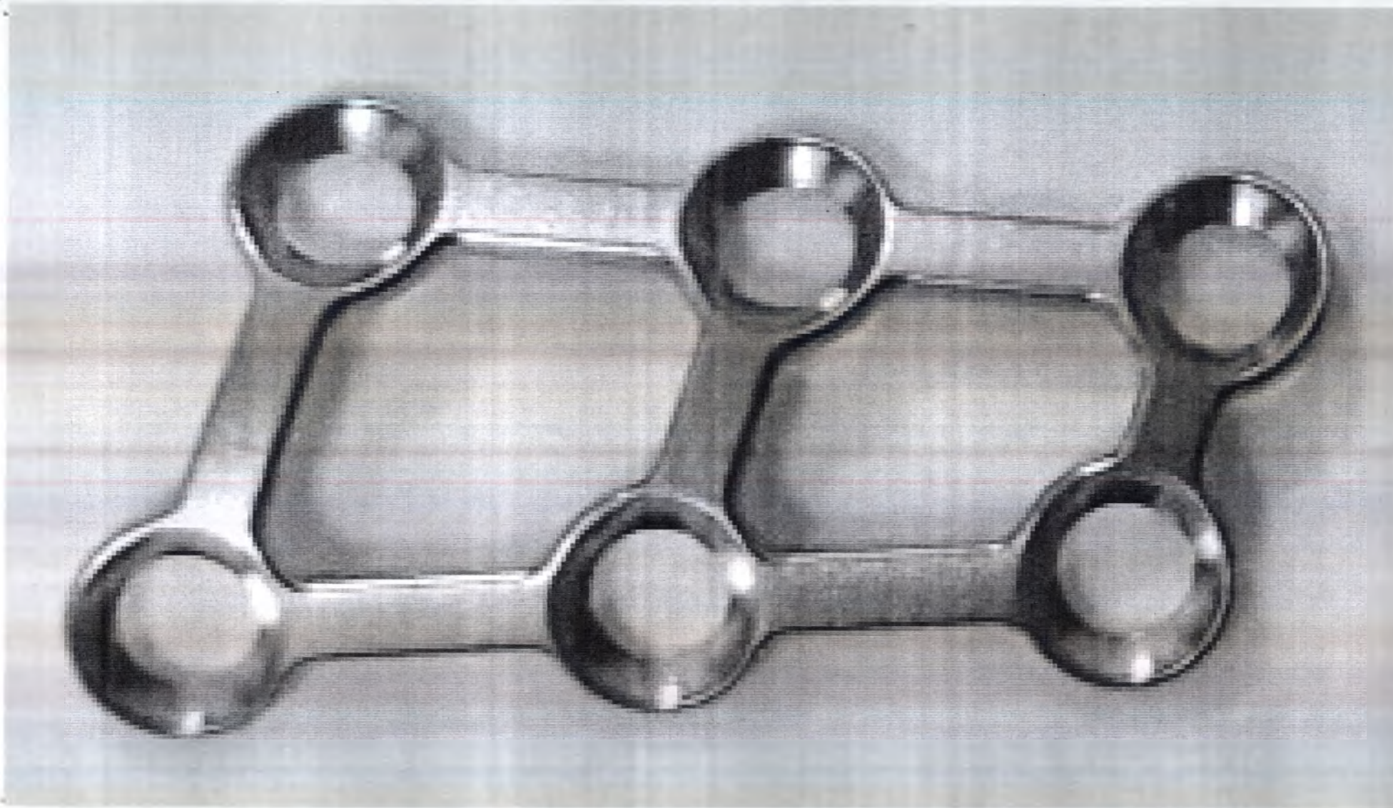
Пластина ARIX Hand System Bone Plate H1-QD-206-L; Внешний вид моделей H1-QD-206-L; H1-QD-206-R идентичен
