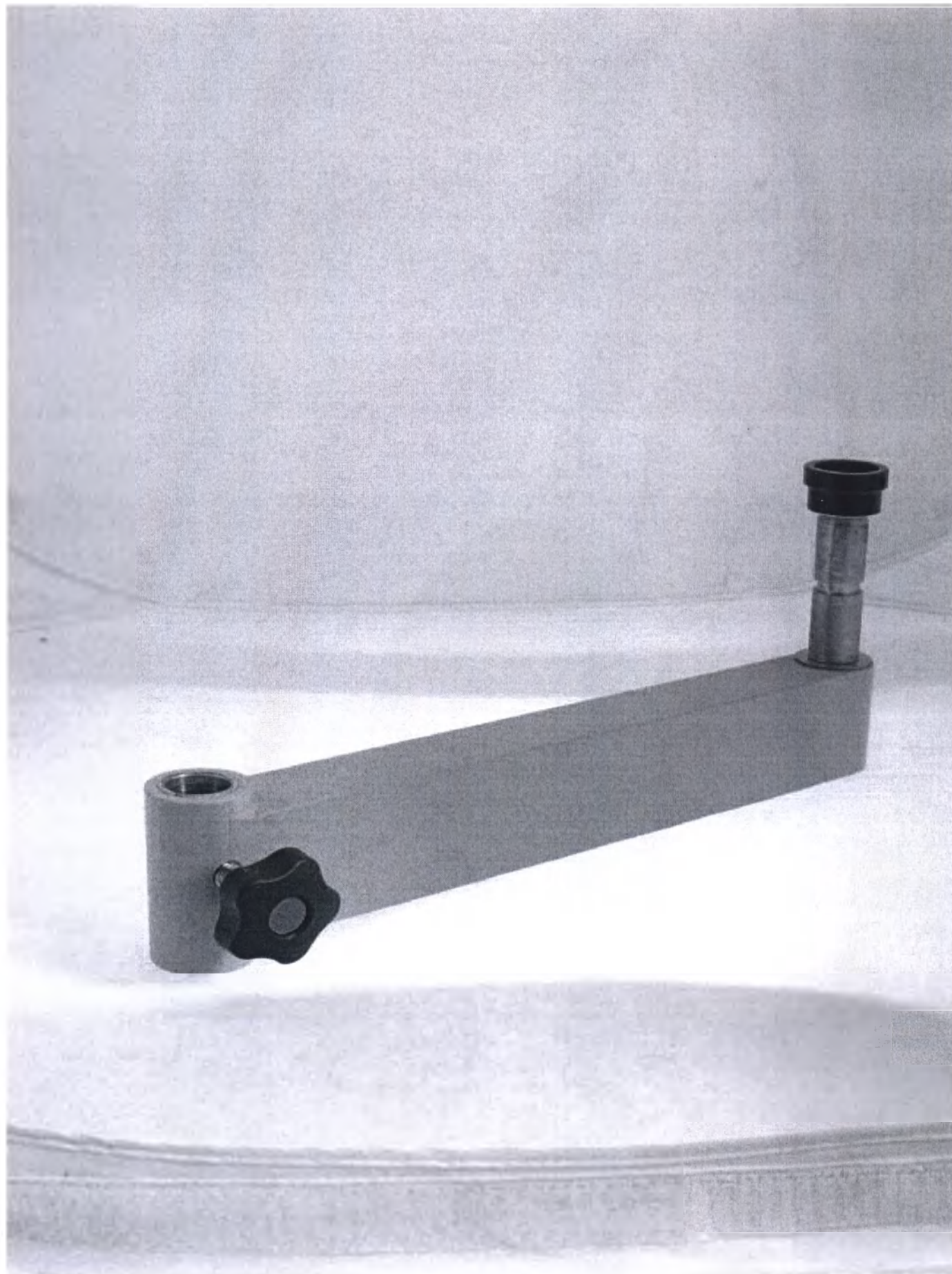
Рис 26. - Удлинитель плеча, длина 28 см;
