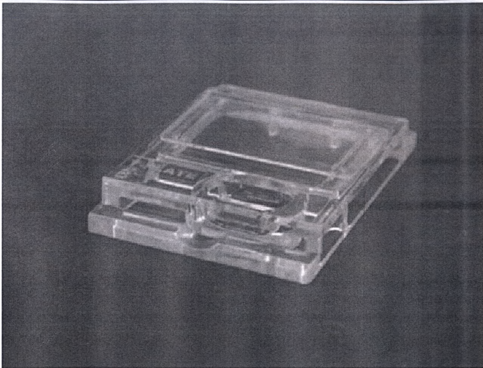
Камера пластиковая T-PLATE для Анализатора автоматического клеточного состава мочи Uscanner (E)
