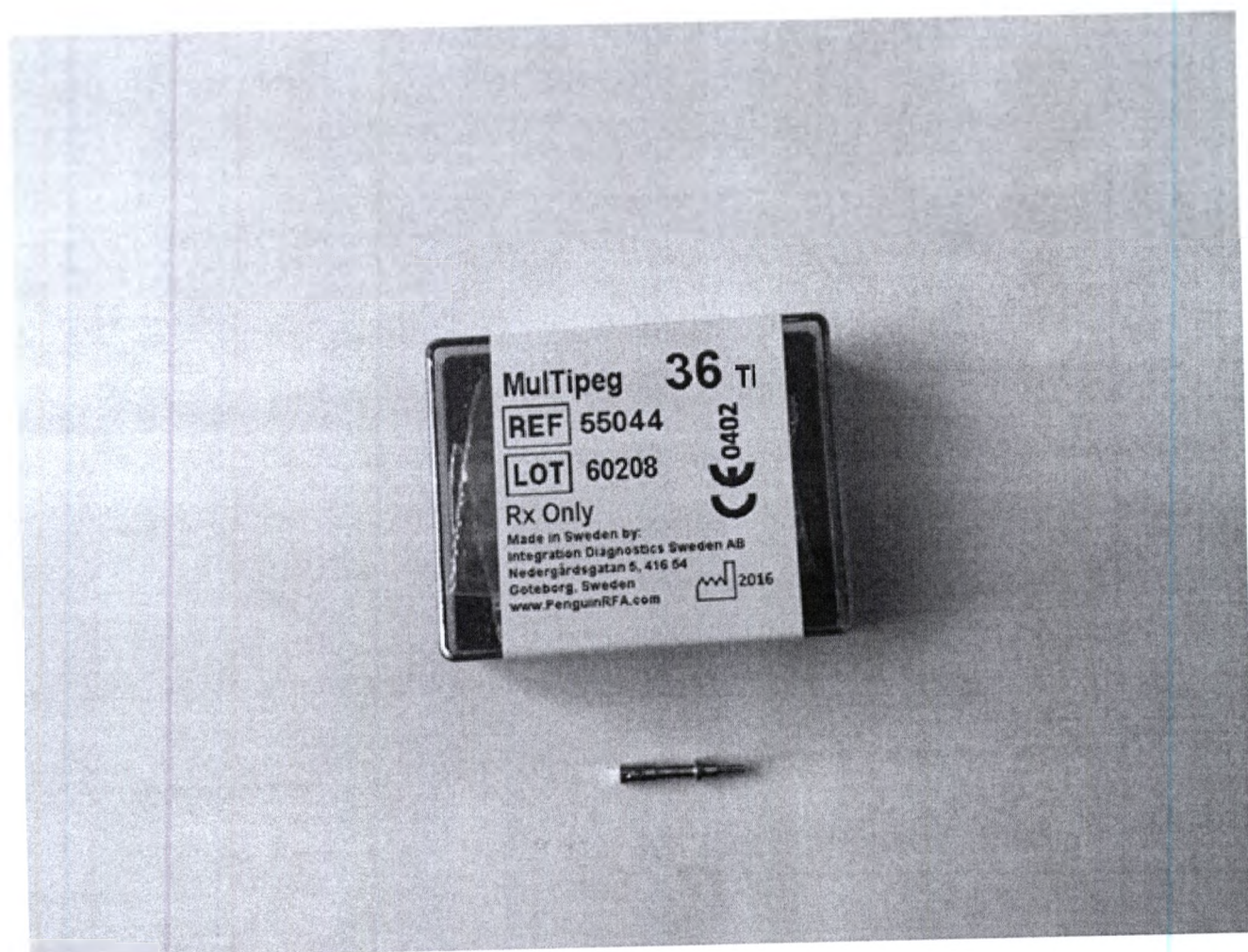
Рис. 36 Штифт MultiPeg 36
