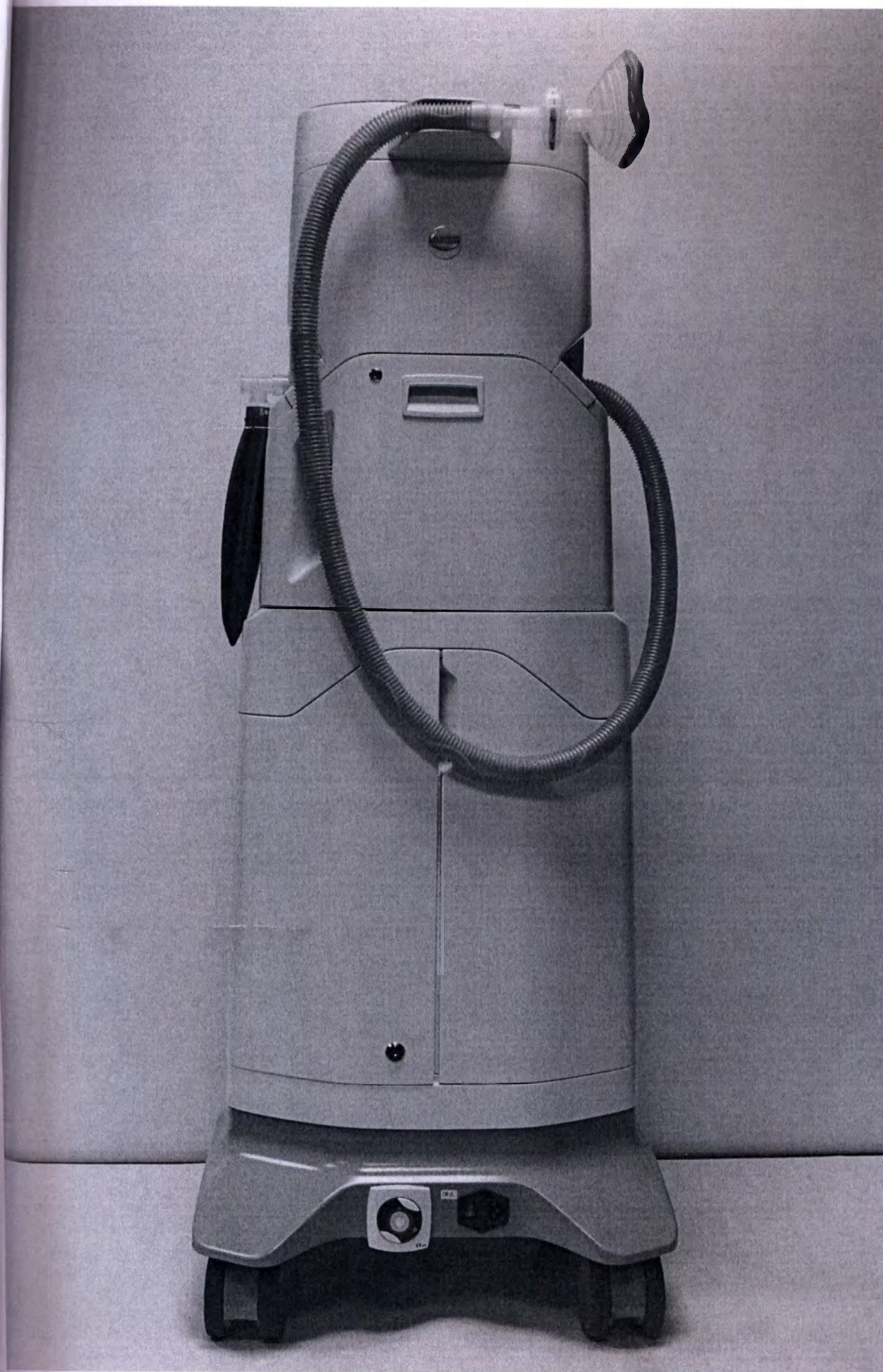
Комплекс терапевтический ксеноновый НОБИЛИС вариант исполнения передвижной, вид сзади
