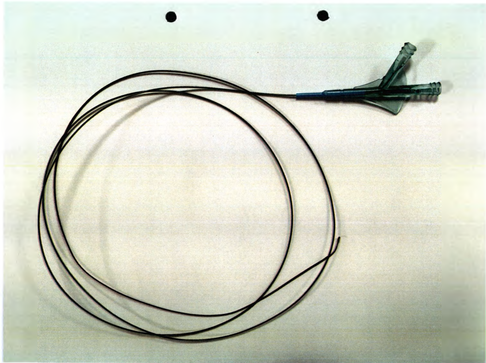
Рис 1.3 Общий вид изделия ECL2L6x12SN
