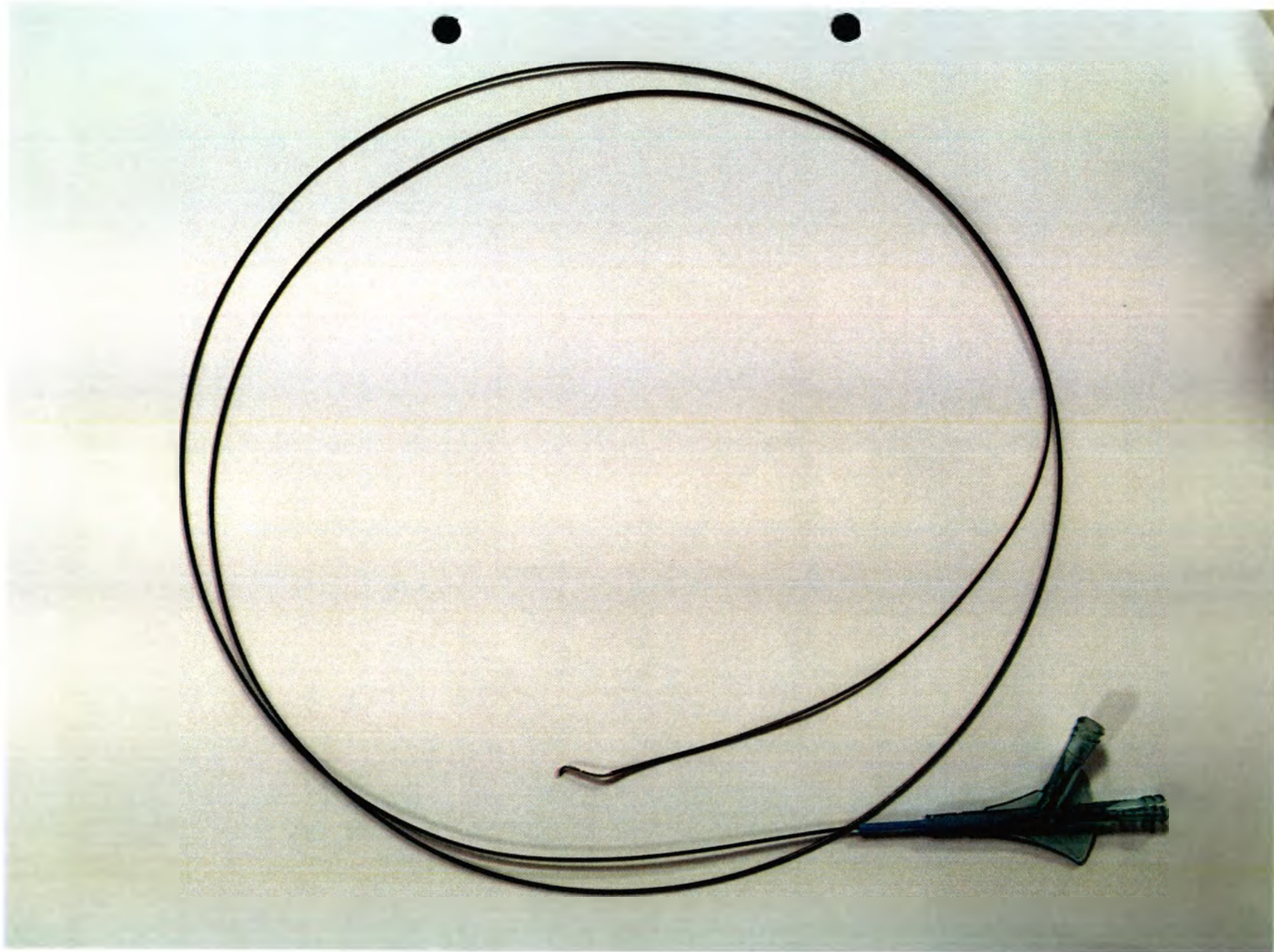
Рис 1.7 Общий вид изделия ECL2L6x9
