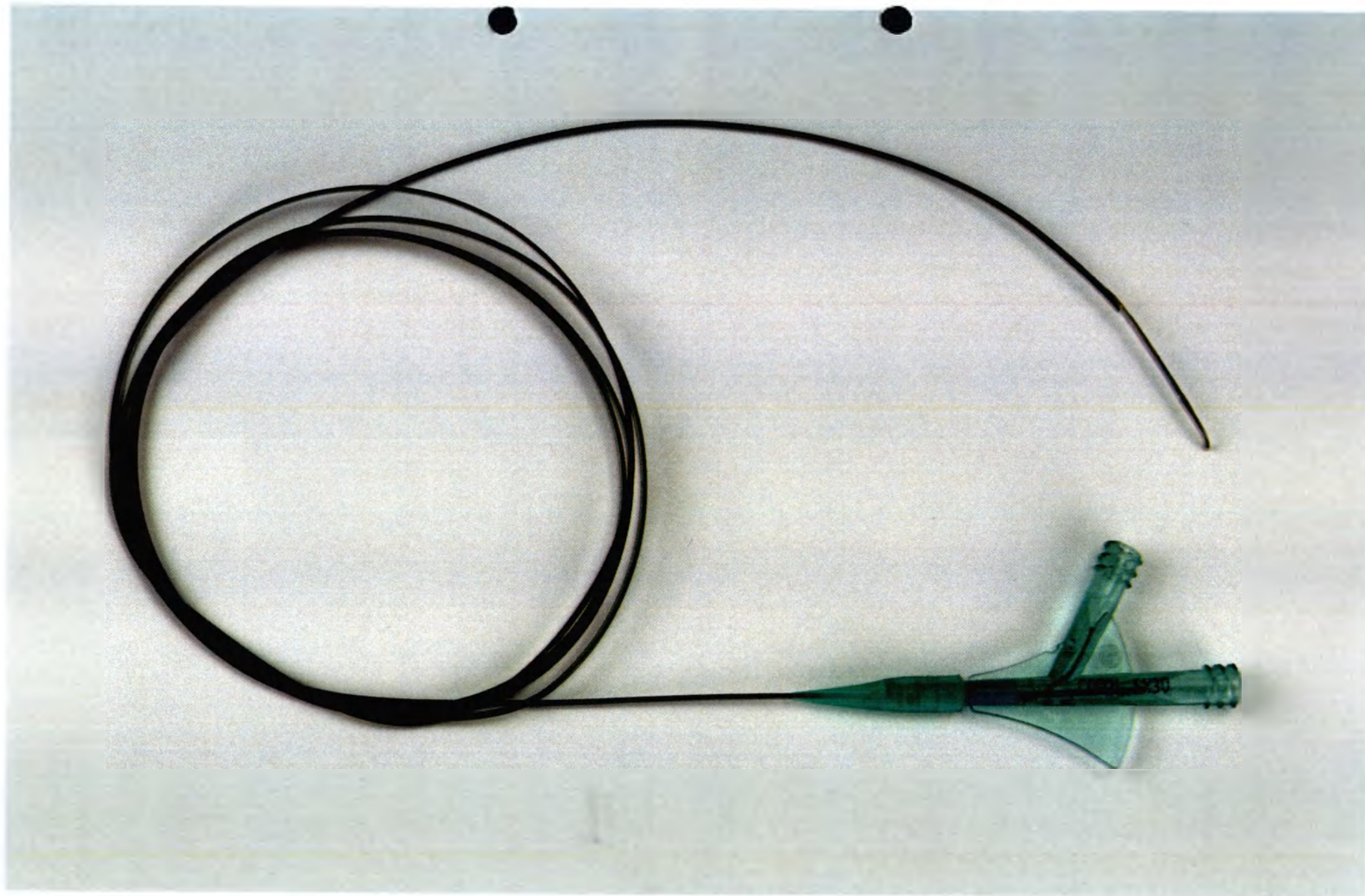
Рис 1.18 Общий вид изделия COP2L6x30
