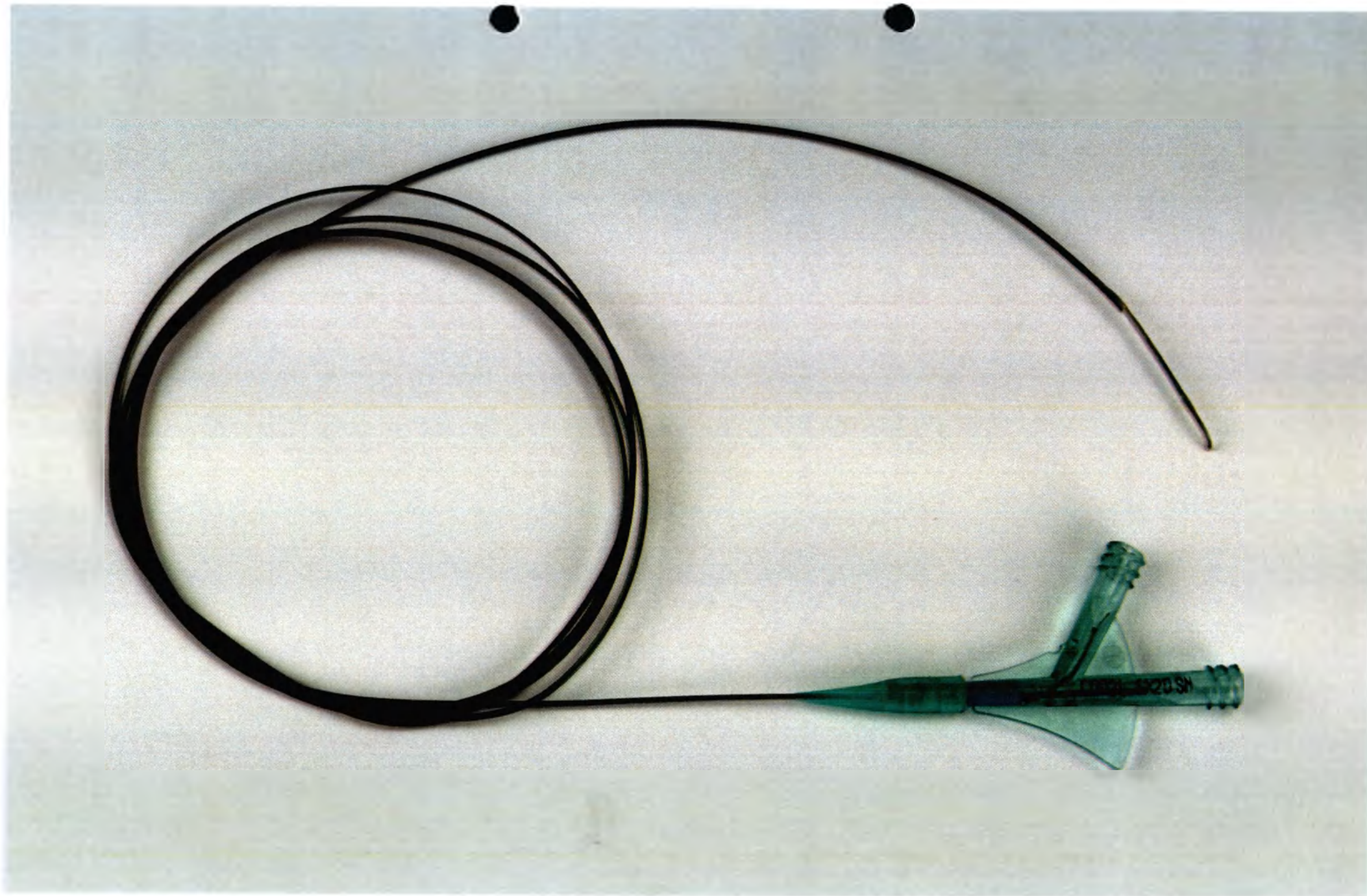
Рис 1.13 Общий вид изделия COP2L6x20SN
