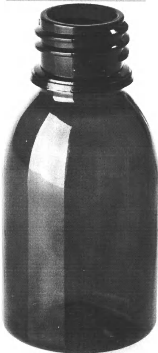
Рисунок 129 – Вариант исполнения: Флаконы из полиэтилентерефталата для лекарственных средств с колпачками № 2 ПЭ 18-Л, 9258. Типоразмер флаконов: флакон ПЭТФ 18/5/25-Л, 1232:
