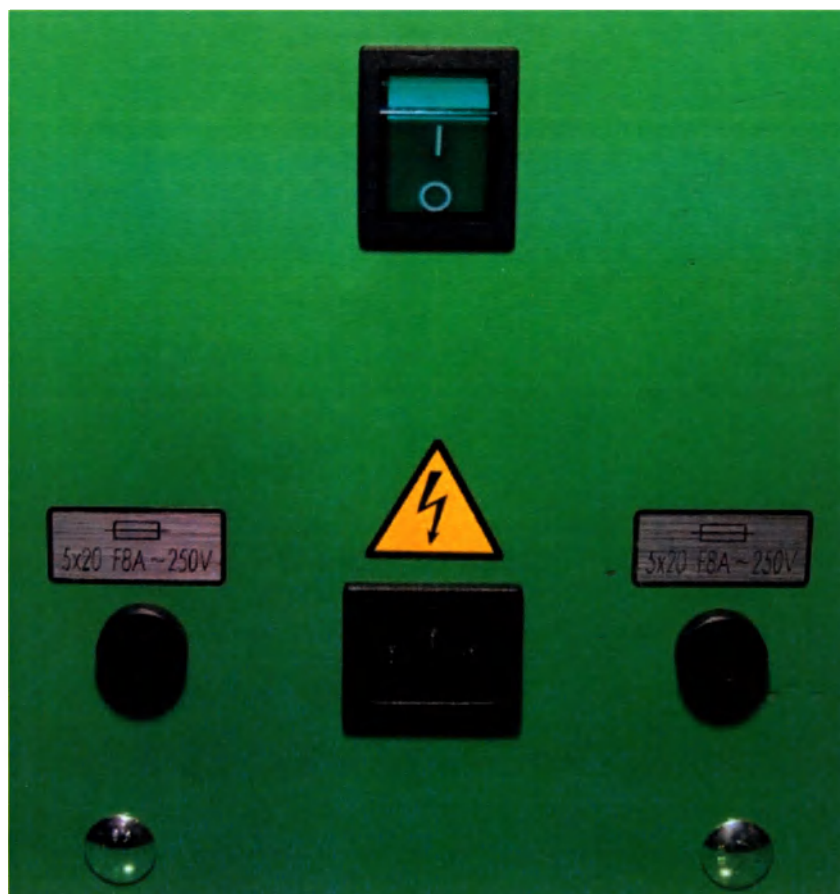
Рис. 2. Сетевой выключатель, гнездо питания, предохранители на задней панели тумбы.
