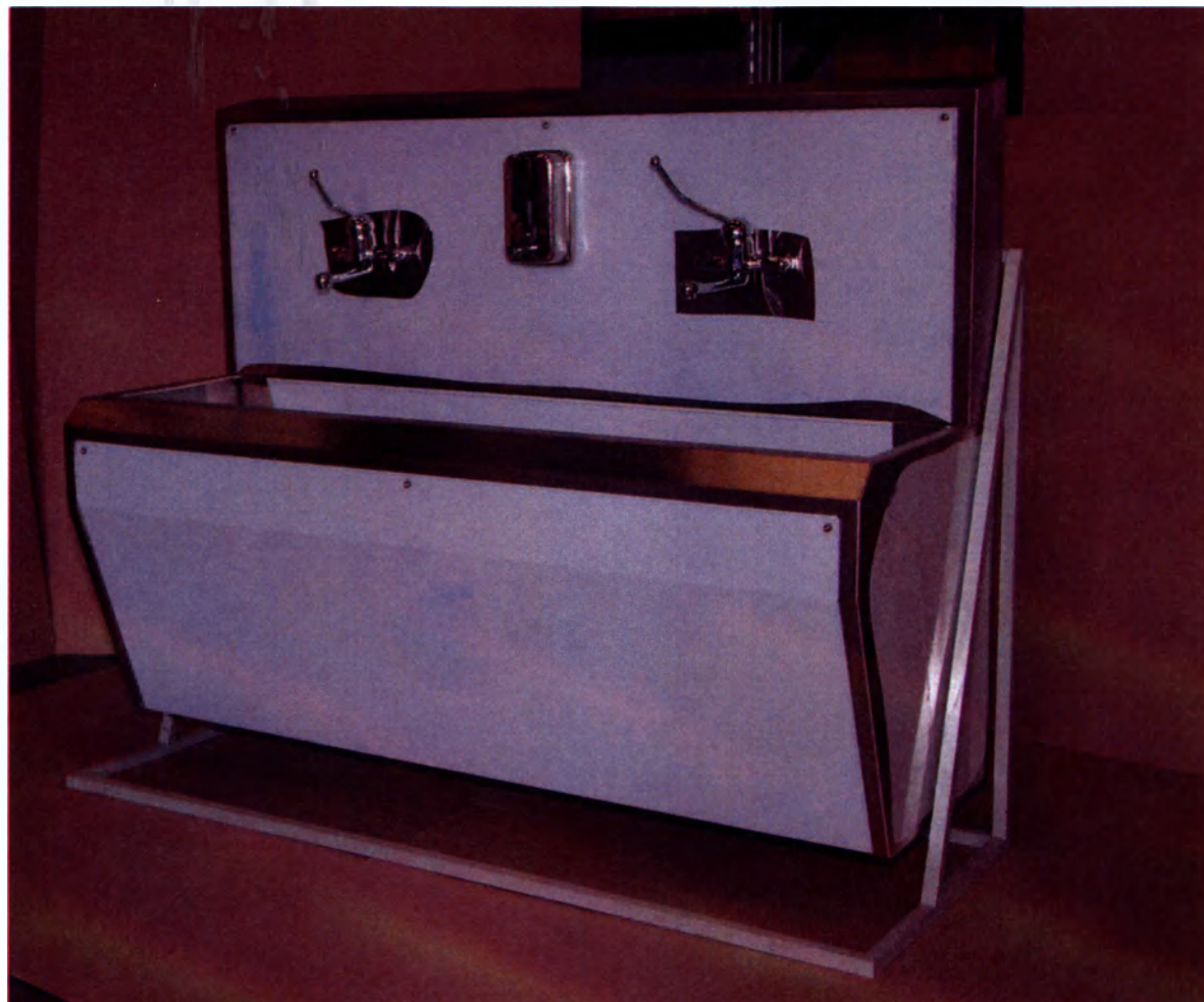
Фото 2. Мойка хирургическая БТ-МХ-2. ТУ 9451-007-99653782-2015
