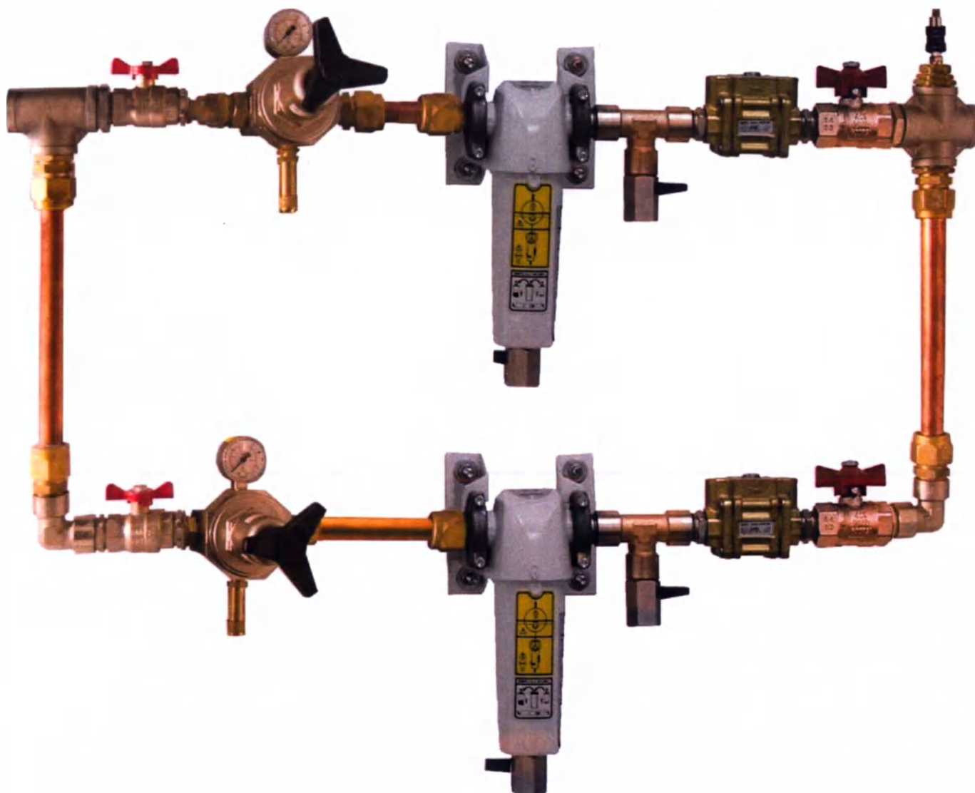
блок окончательной фильтрации и редукции модели DP 434 DP
