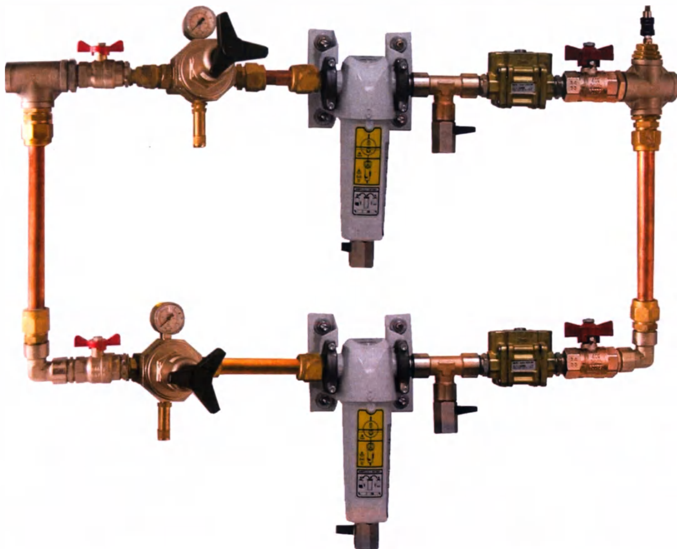
блок окончательной фильтрации и редукции модели DP 792 DP
