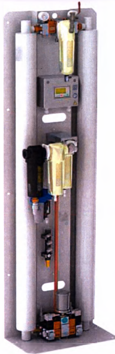
адсорбционный осушитель SEC 7HC модели AD5065
