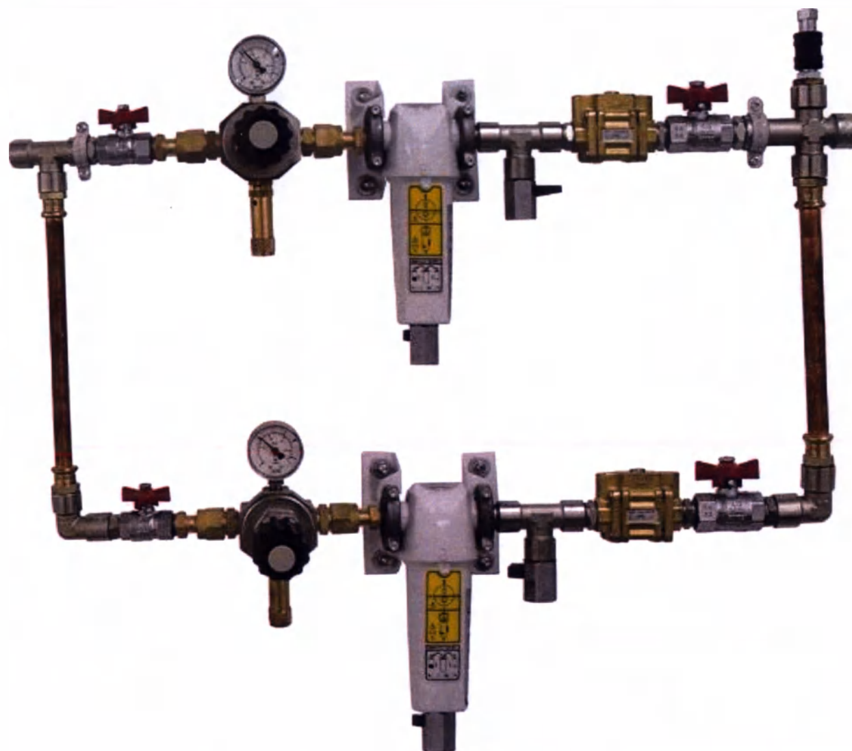
блок окончательной фильтрации и редукции модели DP 72 DP
