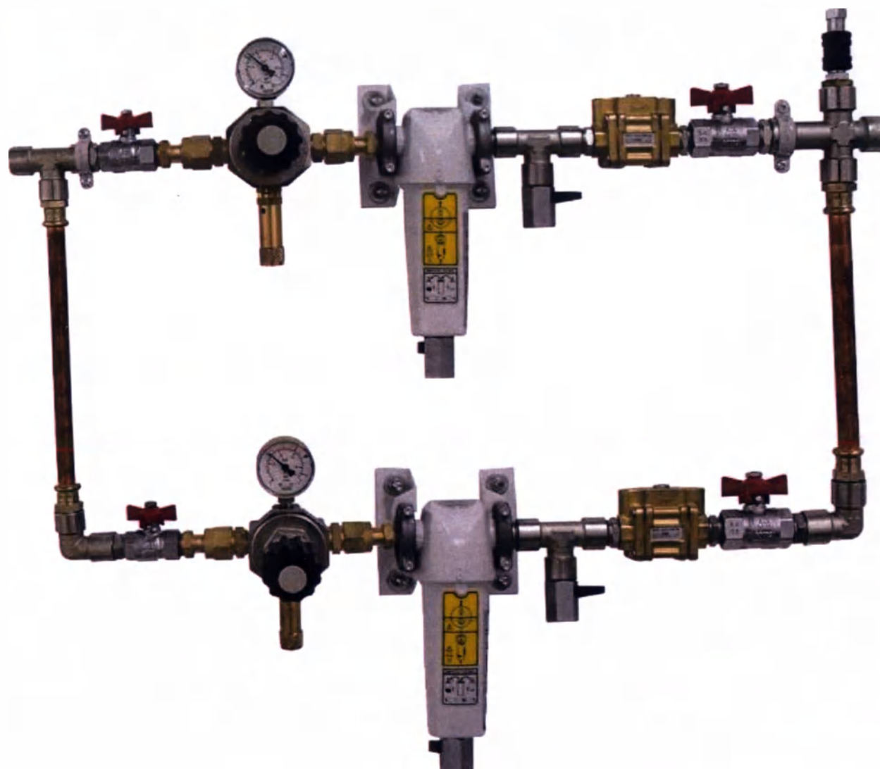
блок окончательной фильтрации и редукции модели DP 144 DP
