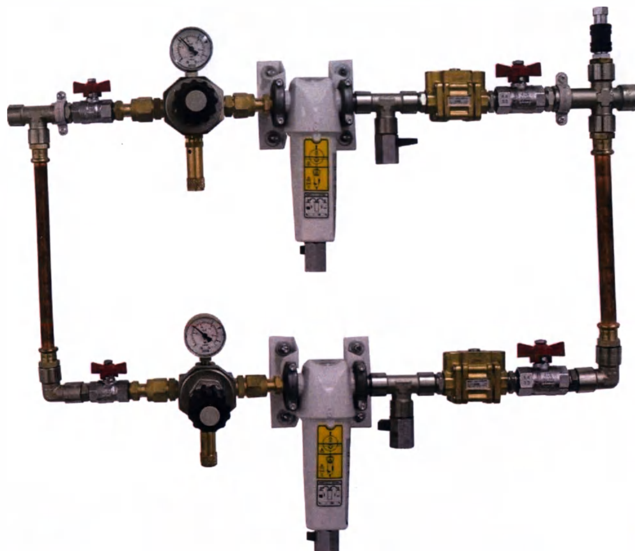
блок окончательной фильтрации и редукции модели DP 218 DP
