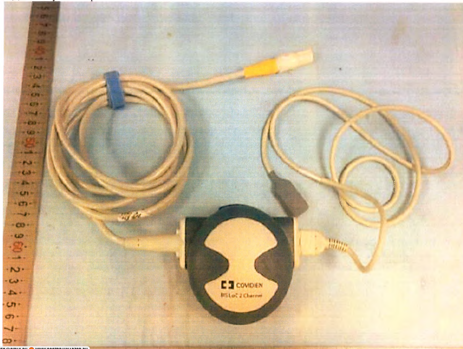
Фото 14. Датчик глубины наркоза
