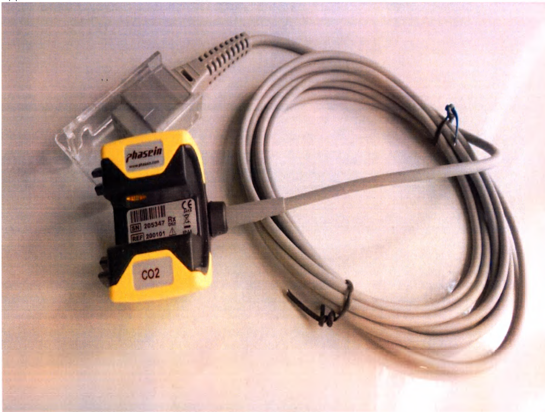
Фото 11. Датчик CO 2
