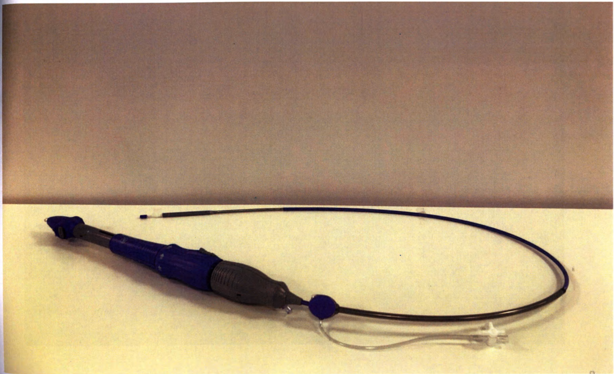
Система катетерной доставки EnVeo R, наружный диаметр 20 Fr (6,7 мм)
