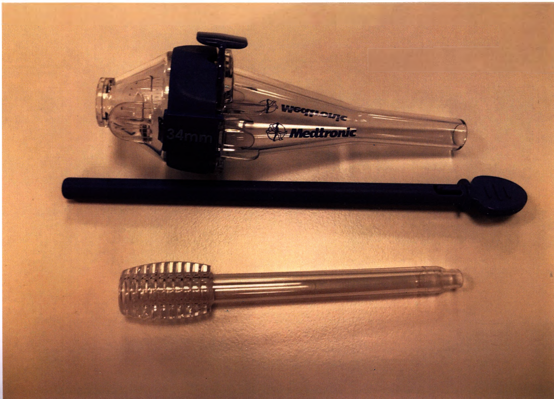
Приспособление для загрузки клапана EnVeo R, размером 34 мм
