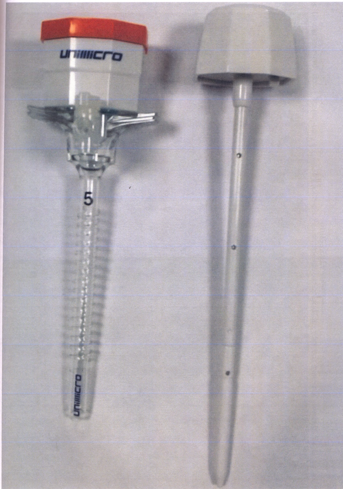
Рис.5 – Троакар хирургический одноразовый с канюлей Hand Pressed Auto-locking Trocar (неразъемный тип) в исполнении ATRHS0507
