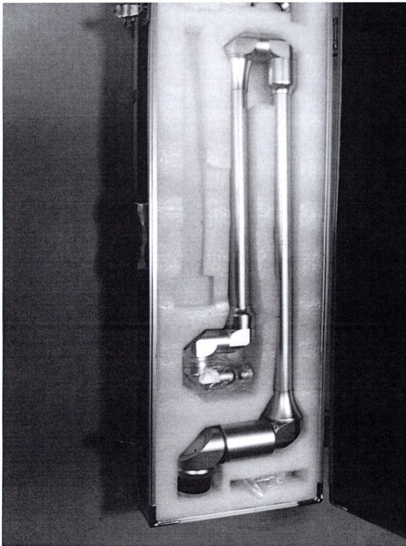
Манипулятор 13 (Тип Б)
