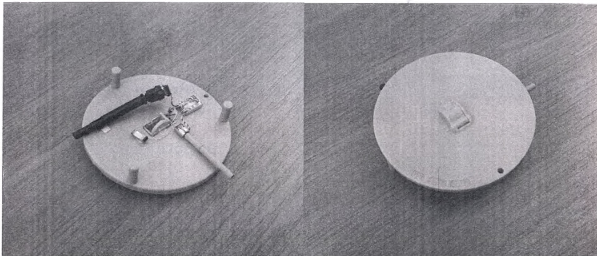
Фейсплата для изготовления индивидуального внутриушного слухового аппарата (вид сверху, вид снизу)
