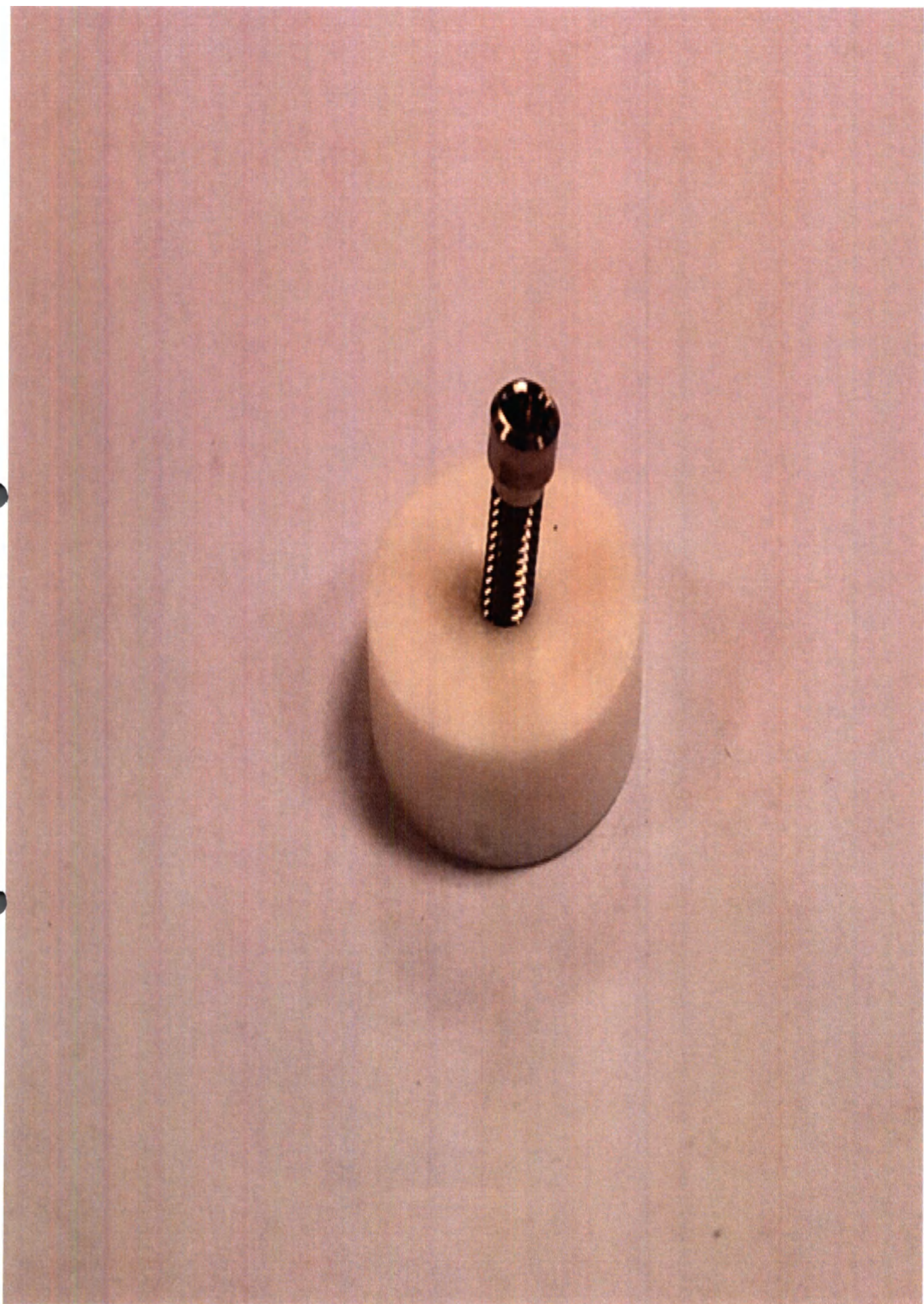
винт фиксирующий позолоченный: TP00-AU, TP01-AU (при необходимости);
