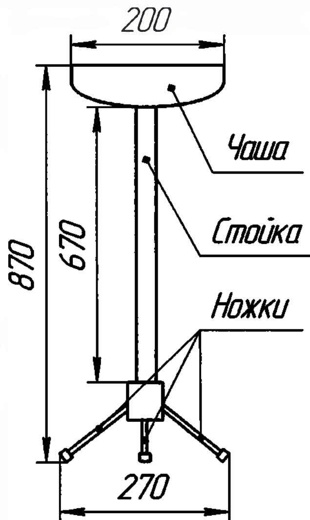
Рис. В.5 - Плевательница стоматологическая
