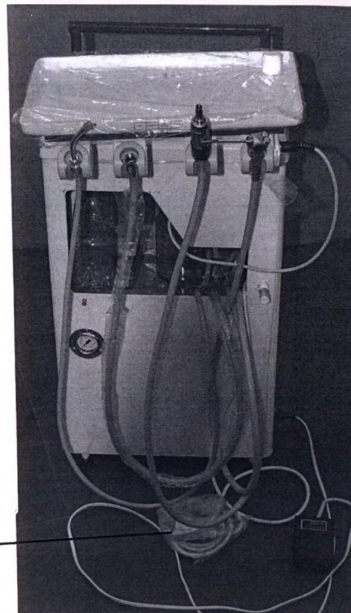
Модуль врача переносной УС-01П
