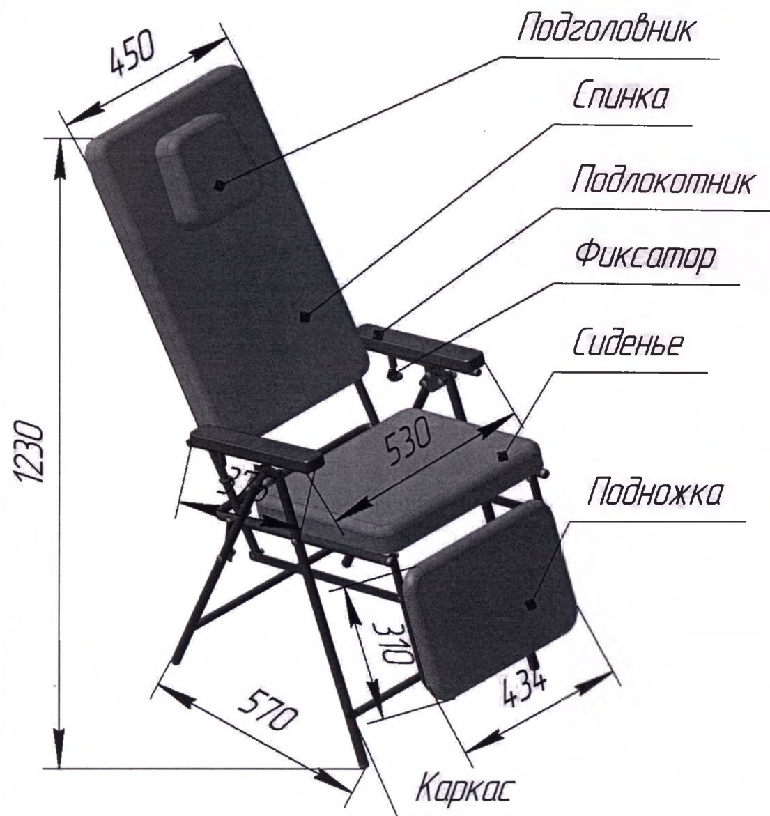
Рис. В.2 – Кресло стоматологическое облегченное
