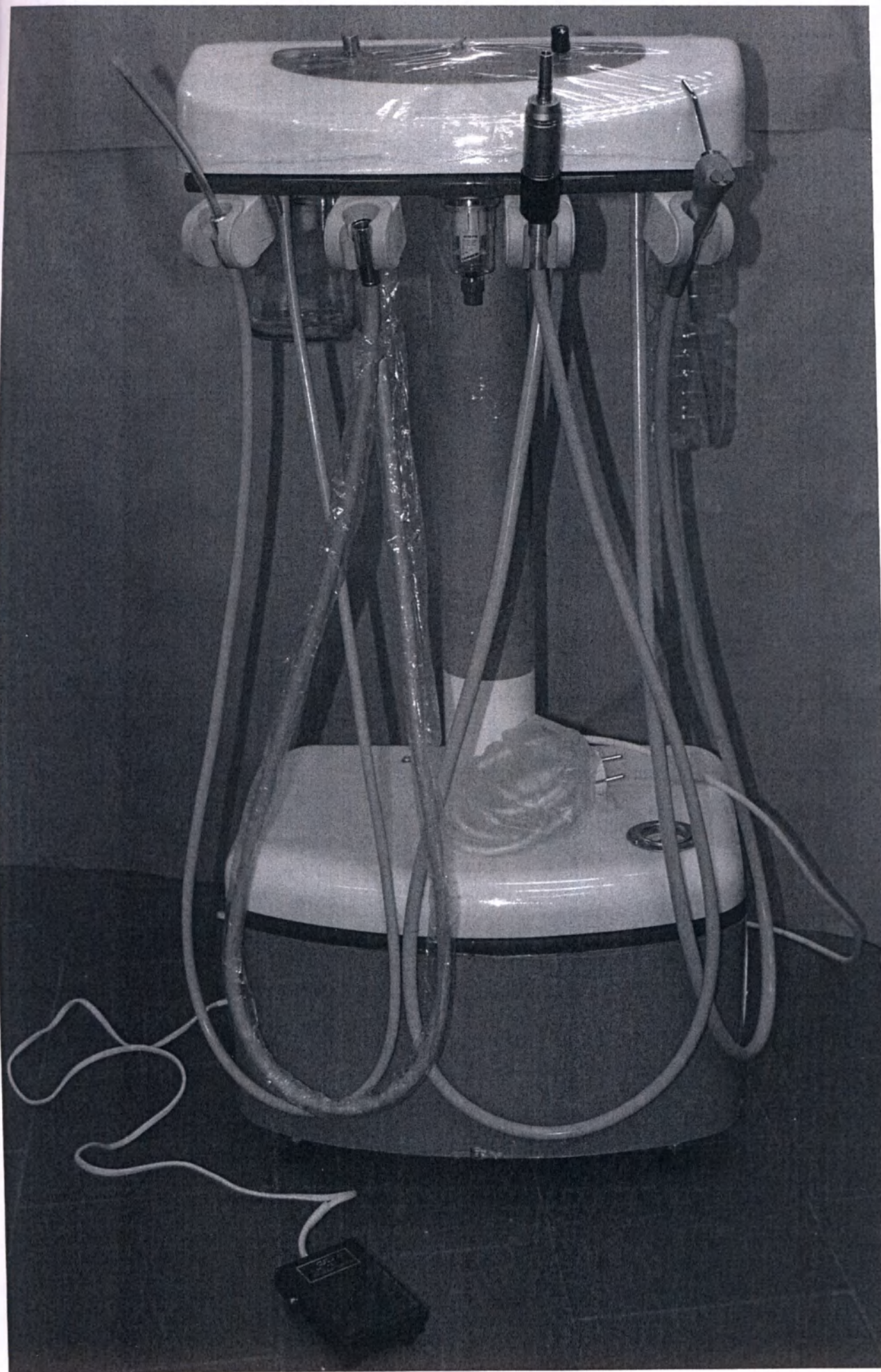
Модуль врача мобильный УС-01М
