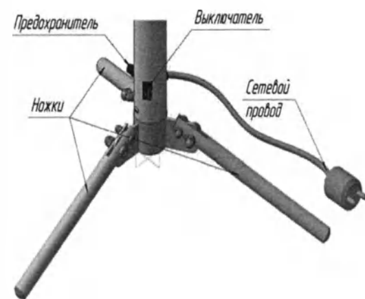
Рис. В.3 - Светильник стоматологический переносной
