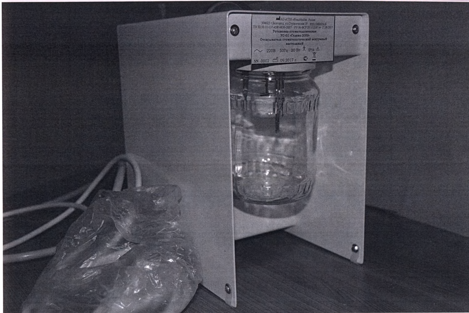
Отсасыватель стоматологический вакуумный настольный (задняя стенка)
