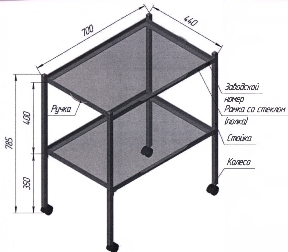
Рис. В.4 - Стол стоматологический инструментальный
