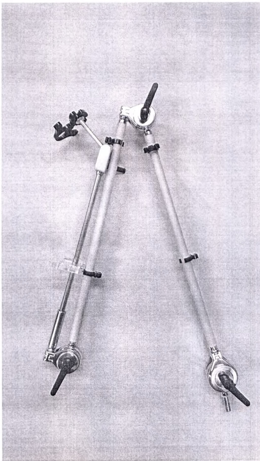
Держатель шлангов
