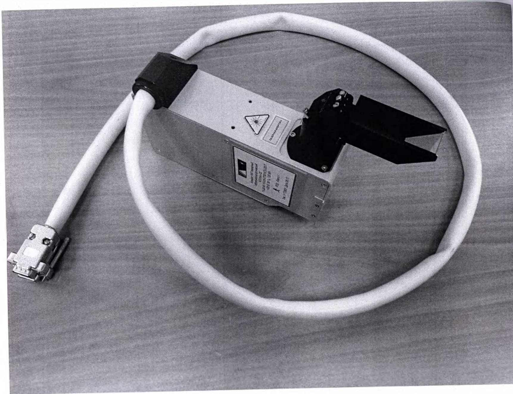
Блок оптический аппарата с соединительным кабелем
