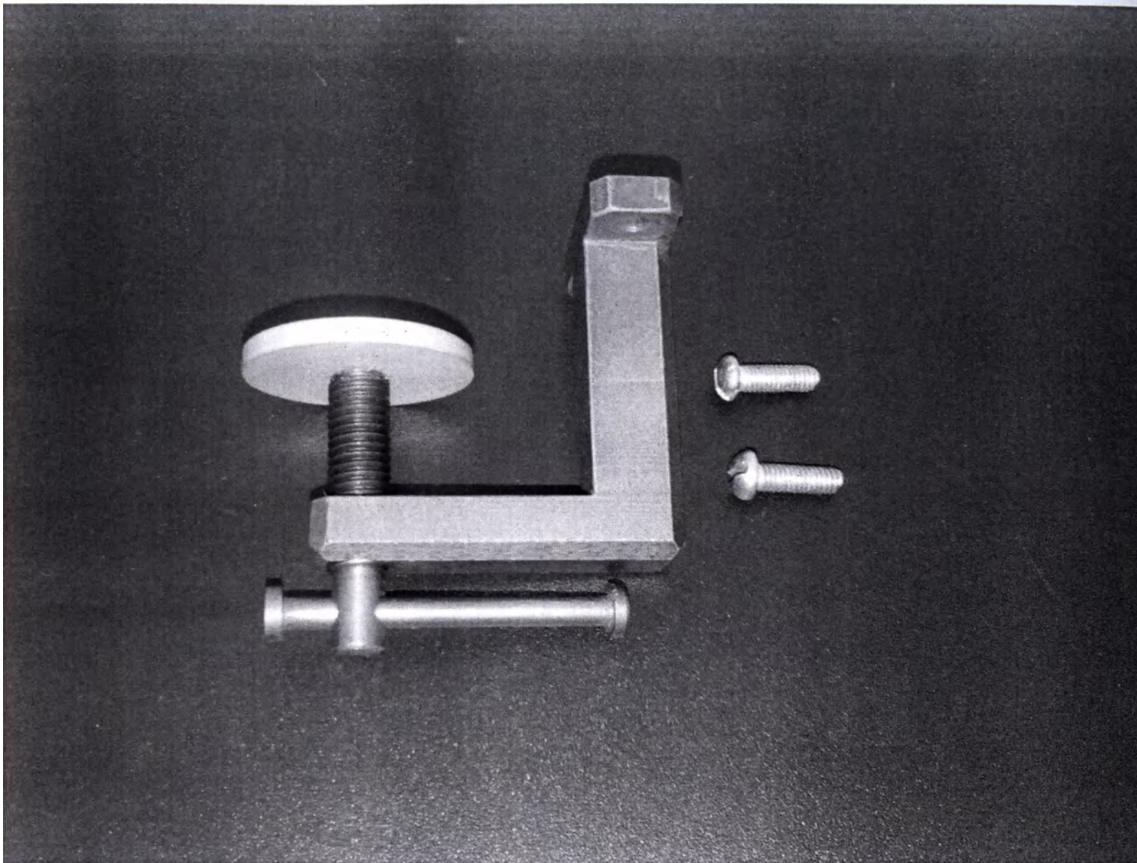
Струбцина крепления к столу блока питания и управления (с винтами)
