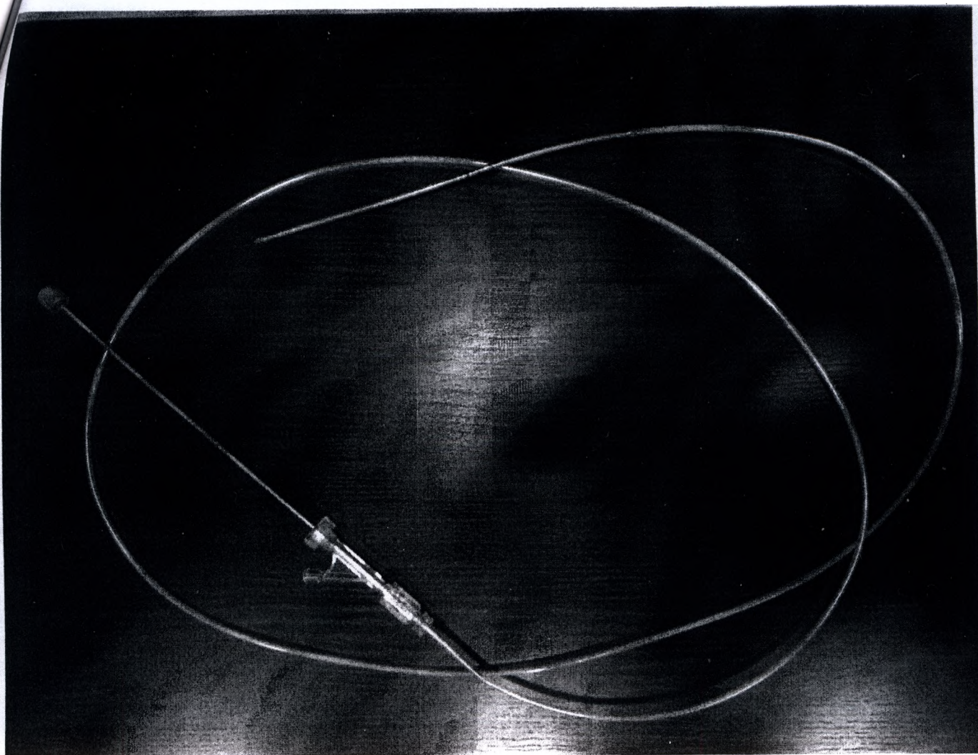
Рисунок 1. Стент мочеточниковый URS с системой доставки URS-A-10-100
