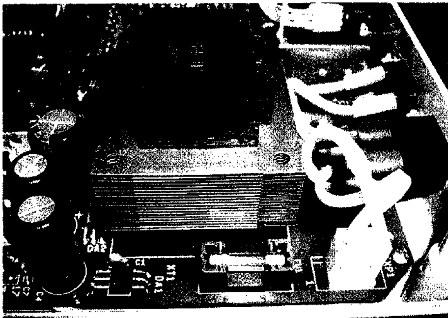
Сетевой трансформатор и плавкий предохранитель
