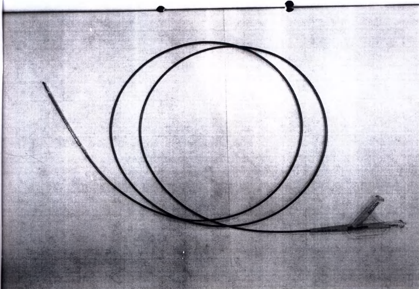
Система для стентирования периферических сосудов Visi-Pro с баллонорасширяемым стентом (общий вид системы доставки со стентом)
