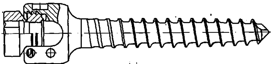
Рисунок А16 - Пример винта моноаксиального
