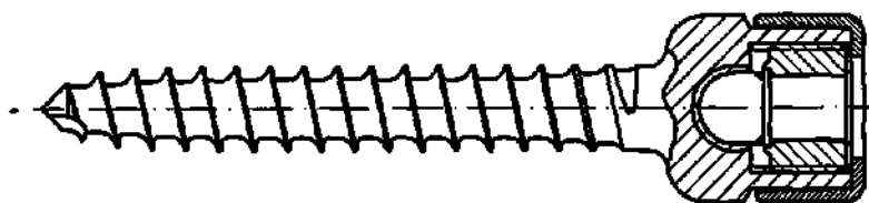
Рисунок А12 - Пример винта пояснично-крестцового
