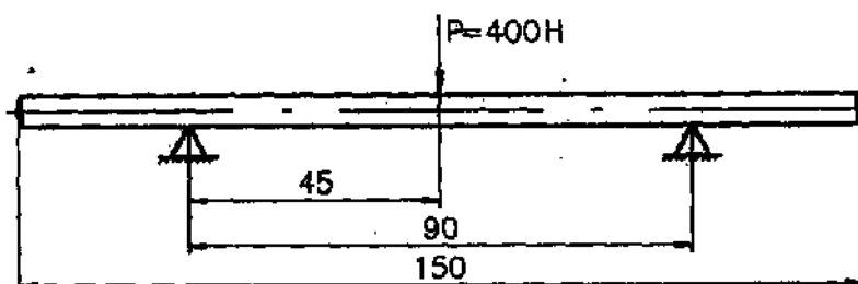
Рисунок Б2 – Схема приложения нагрузок к стержню
