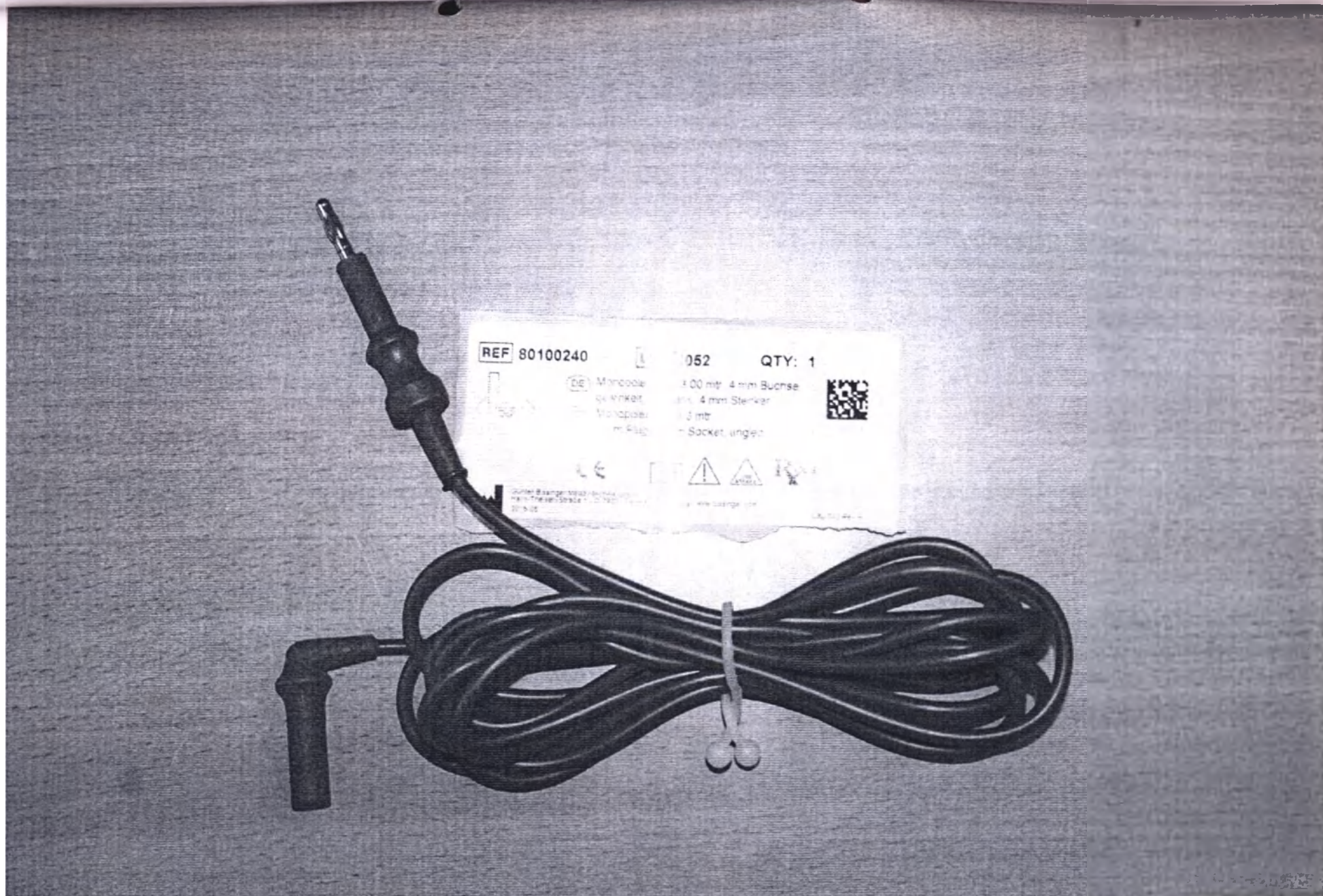
Кабель монополярный со стороны инструмента- плоский Ø 4мм угловой штекер совместимый с генераторами Erbe T-Serie, Martin, Berchtold, 3 м, 80100240. Внешний вид
