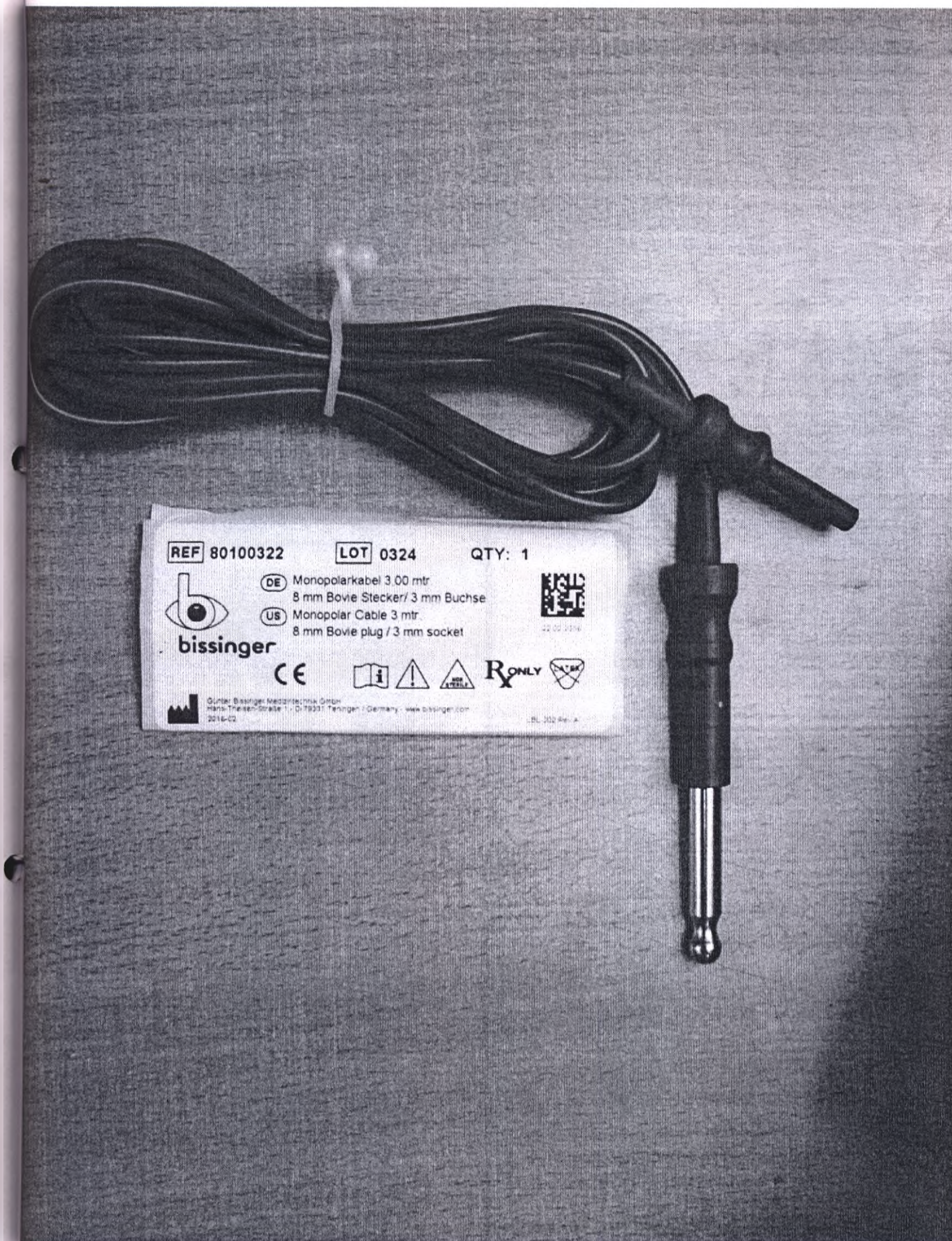
Модель монополярный со стороны инструмента - штекер Ø 3мм совместимый с генератором Bovie, Valleylab, Conmed, 80100322, 3
